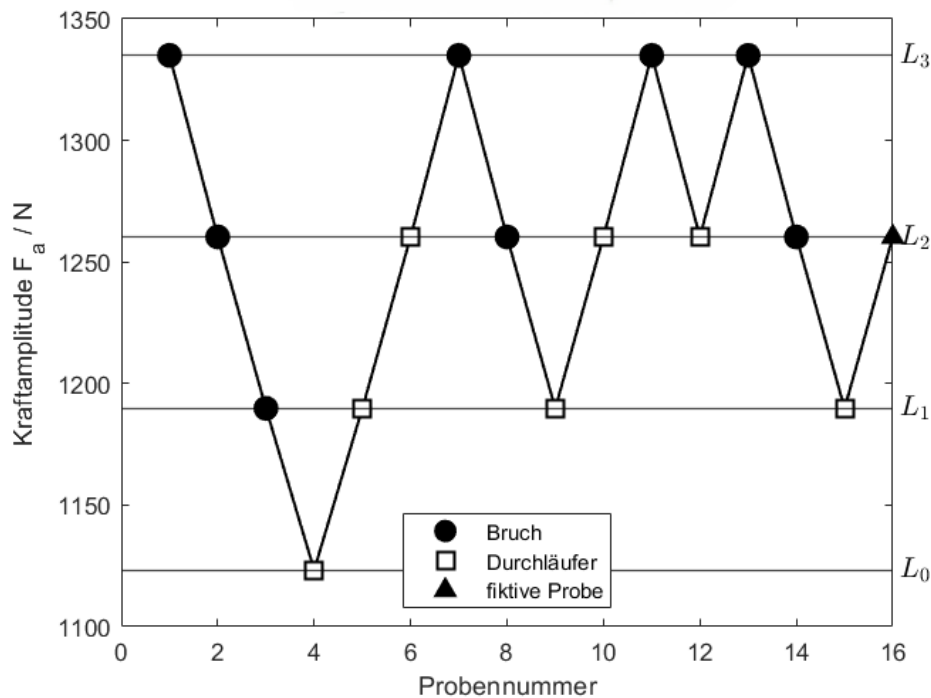
Abbildung 4.7.: Folge im Treppenstufenverfahren.
