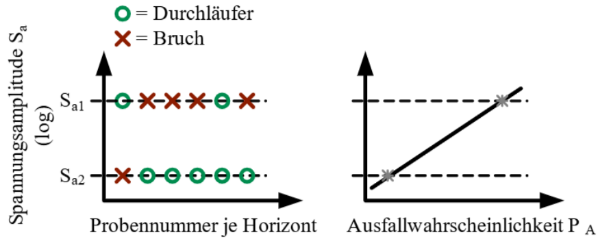
Abbildung 2.12.: Abgrenzungsverfahren [18, Seite 33].
