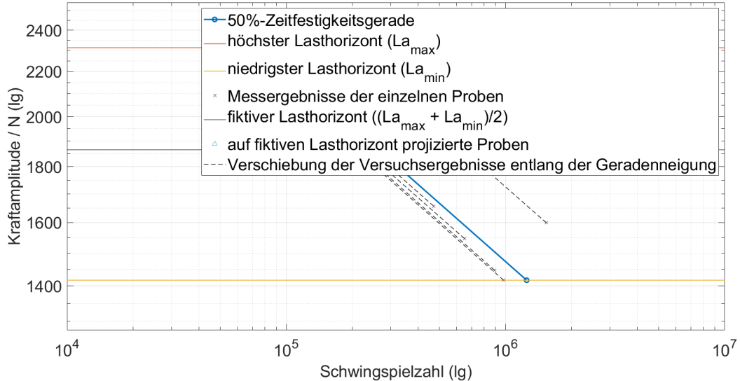
Abbildung 4.6.: Verschieben der Versuchsergebnisse auf einen gemeinsamen Lasthorizont (In Anlehnung an DIN 50100, Seite 56).
