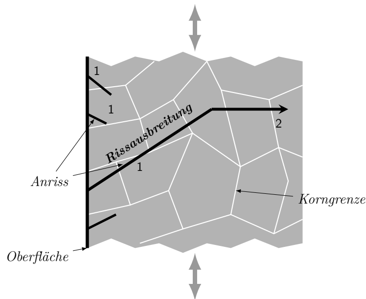
Abbildung 2.2.: Risstadium 1 und 2 (In Anlehnung an [8, Seite 212]).
