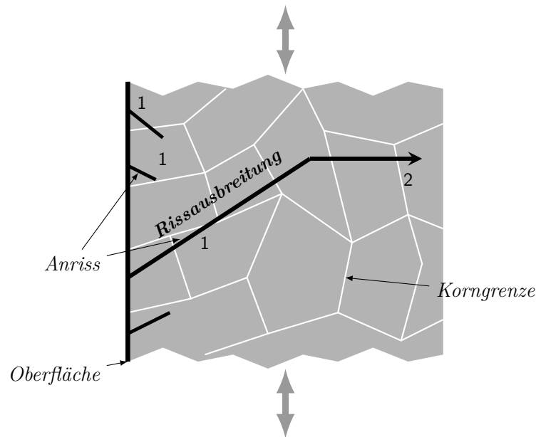
Abbildung 2.2.: Rissstadium 1 und 2 (In Anlehnung an [7, Seite 268]).
