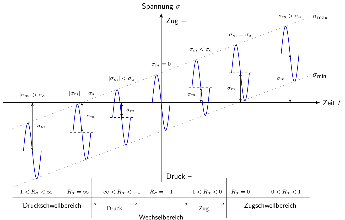
Abbildung 2.4.: Lastfälle schwellend und wechselnd (In Anlehnung an [6, Seite 271], ergänzt um Betragsstriche nach [11, Seite 17]).
