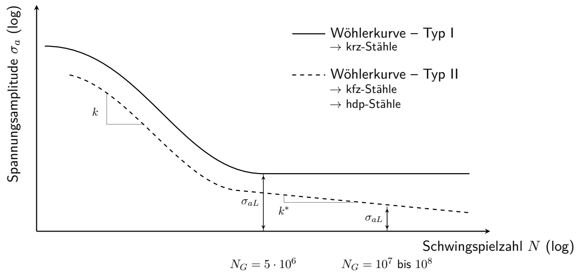
Abbildung 2.7.: Vergleich Typ I und Typ II der Wöhlerkurve.
