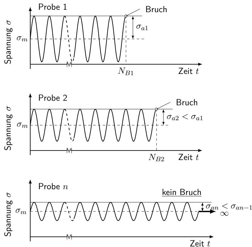
Abbildung 2.5.: Schwingungen der Einzelproben mit gleicher Mittelspannung und unterschiedlicher Spannungsamplitude (eigene Darstellung in Anlehnung an [5, Seite 273]).
