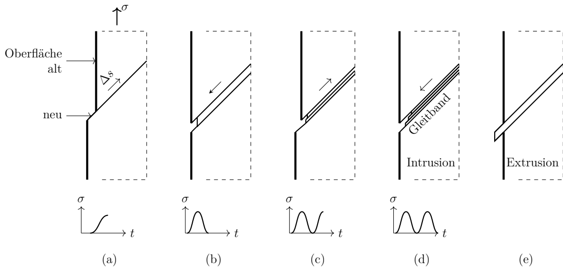
Abbildung 2.2.: Entstehung von Gleitbändern, sowie Intrusionen und Extrusionen infolge zyklischer Beanspruchung (eigene Darstellung in Anlehnung an [10, Seite 8]).
