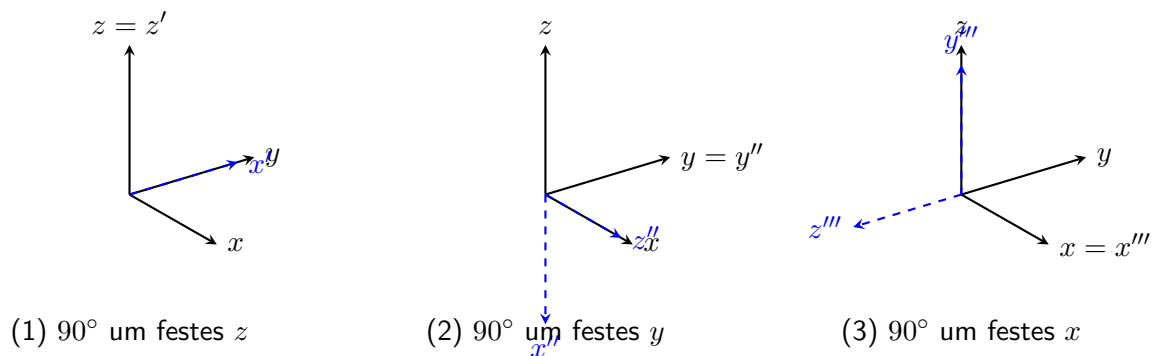
Abbildung 2.8.: Gegenüberstellung bei 90^\circ Rotationen. Man beachte die unterschiedlichen Endlagen der Achsen.
