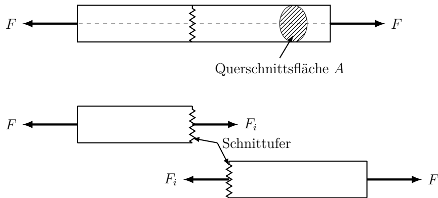
Abbildung 2.1.: Rundstab mit Zugkraft [8, Seite 202].
