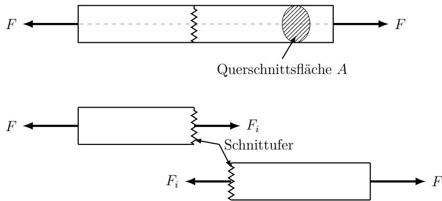
Abbildung 2.1.: Rundstab mit Zugkraft [11, Seite 202].
