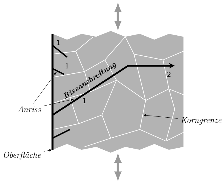
Abbildung 2.2.: Rissstadium 1 und 2 (In Anlehnung an [8, Seite 268]).
