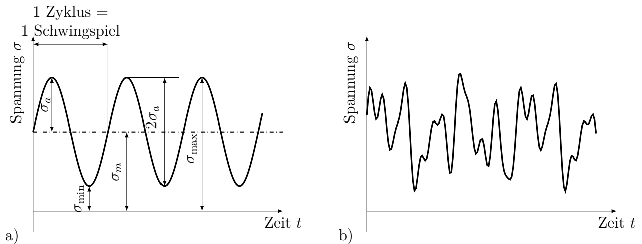
Abbildung 2.3.: Lastzeitverläufe: a) Kenngrößen am Beispiel einer periodischen Sinusschwingung, b) stochastische Betriebslast (In Anlehnung an [8, Seite 269-270]).
