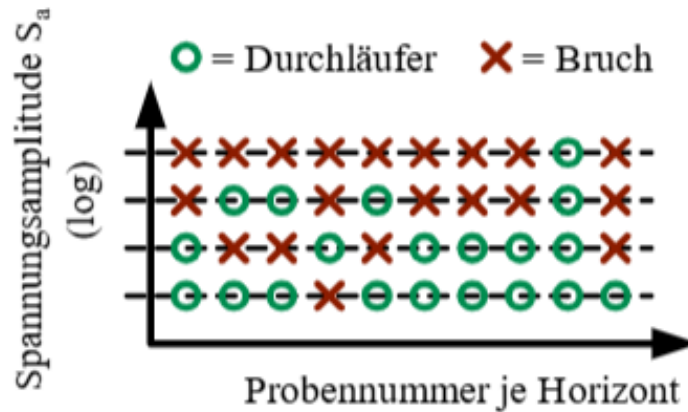
Abbildung 2.11.: Probit-Verfahren [17, Seite 36].
