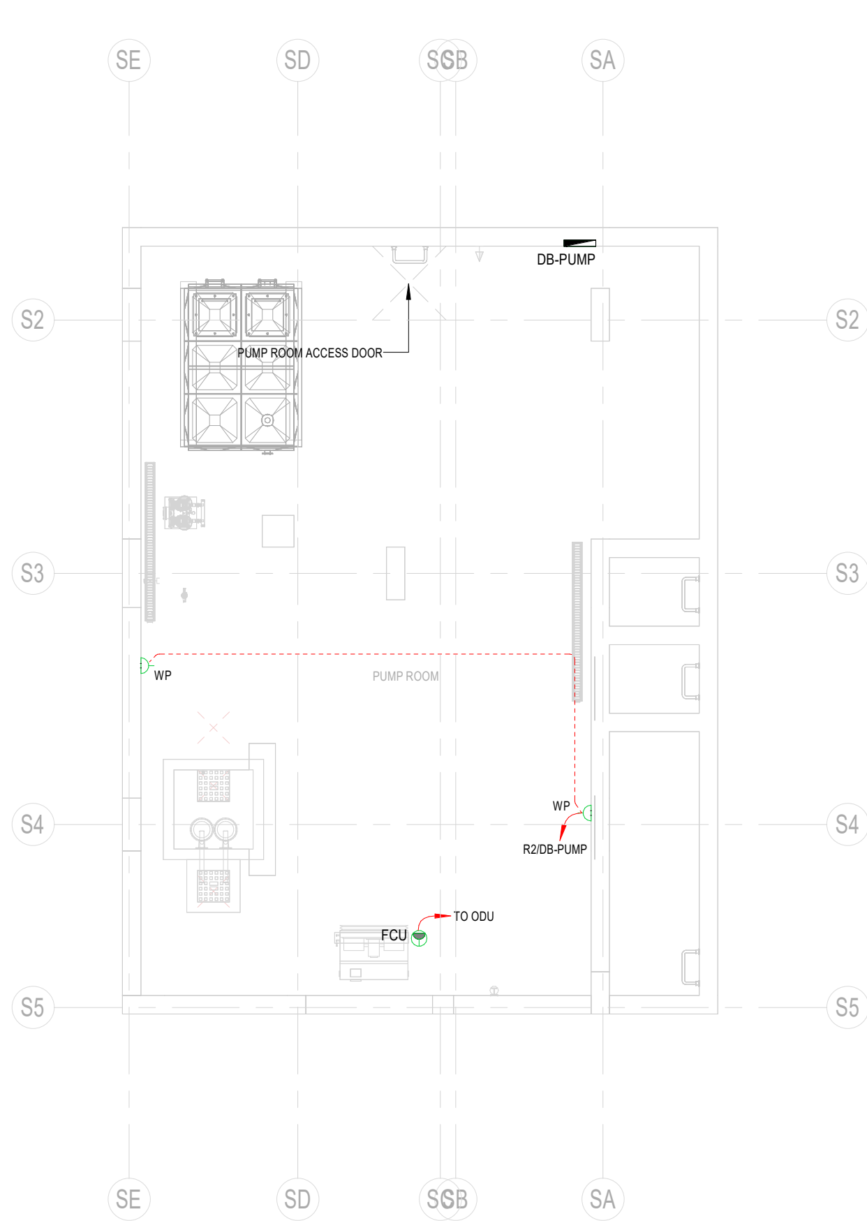
1 00-U.W.T SERVICE BLOCK POWER 1 : 100
