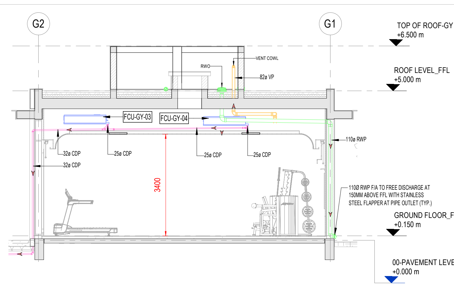
4 GYM&YOGA DRAINAGE SECTION 02 1 : 75
