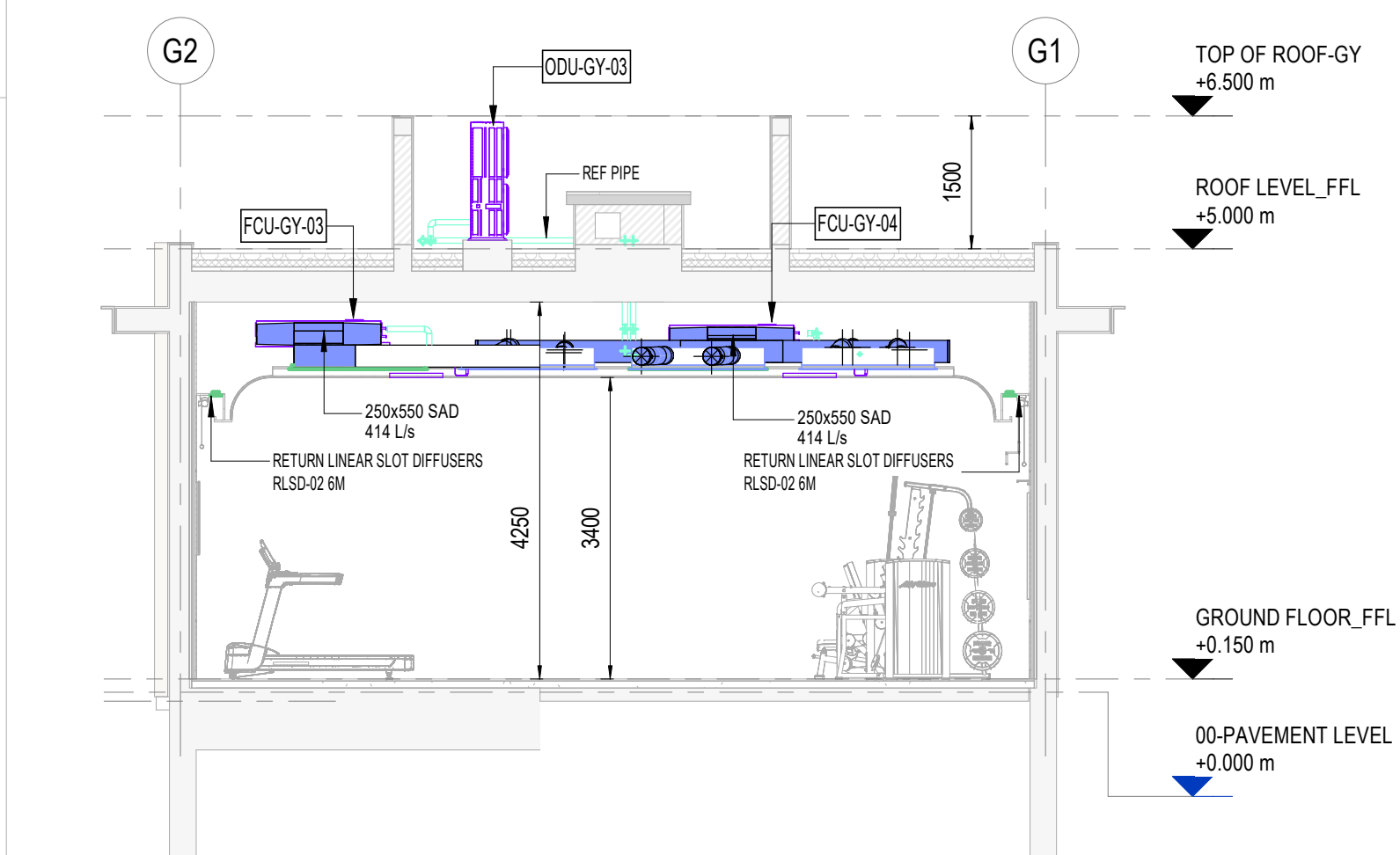
4 GYM&YOGA AC SECTION 02 1 : 75
