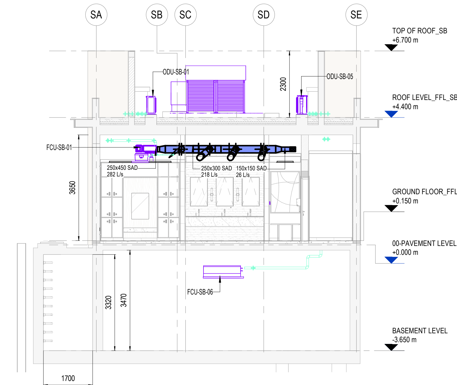
4 SERVICE BLOCK AC SECTION 01 1 : 75
