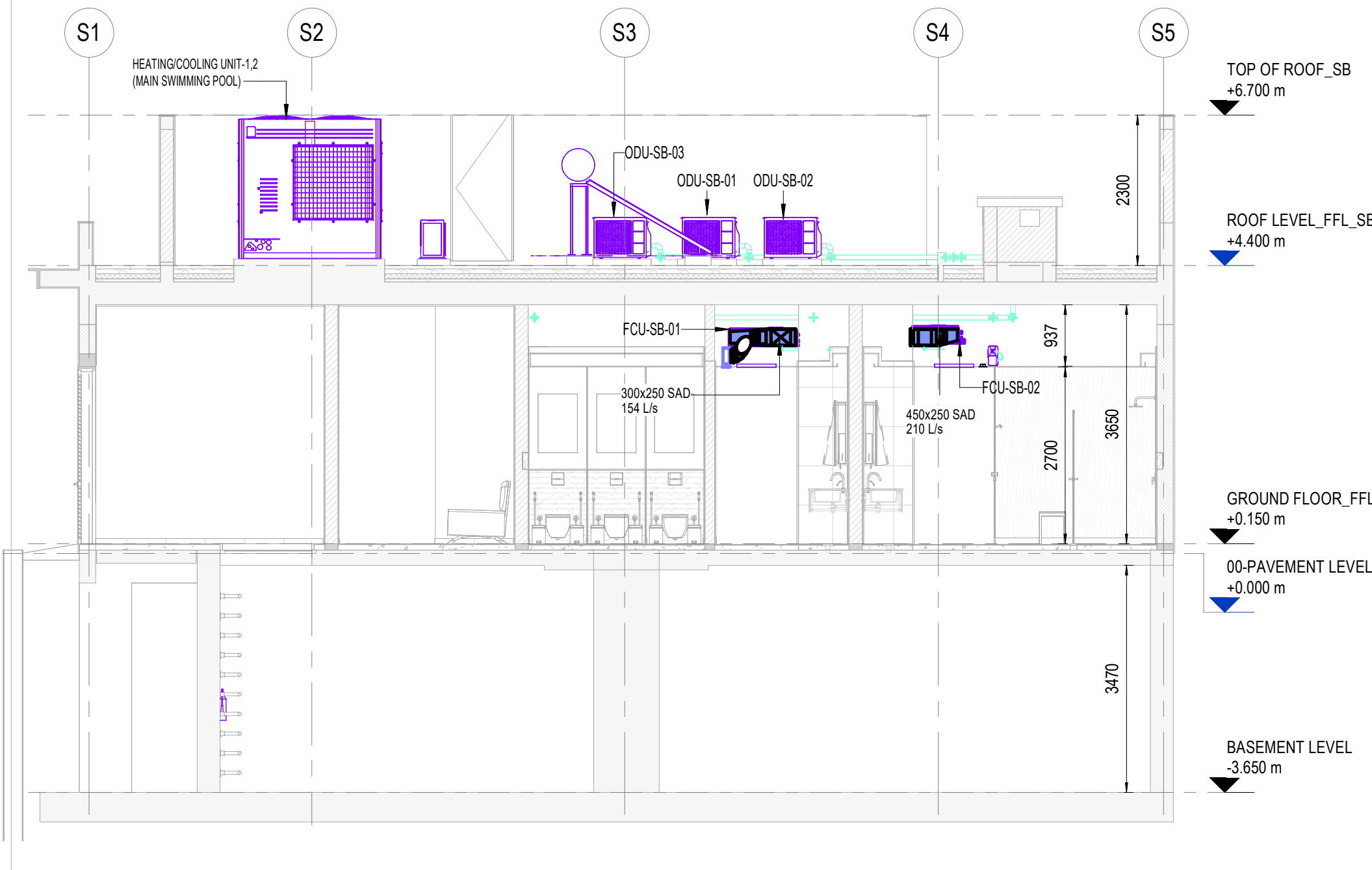
5 SERVICE BLOCK AC SECTION 02 1 : 75
