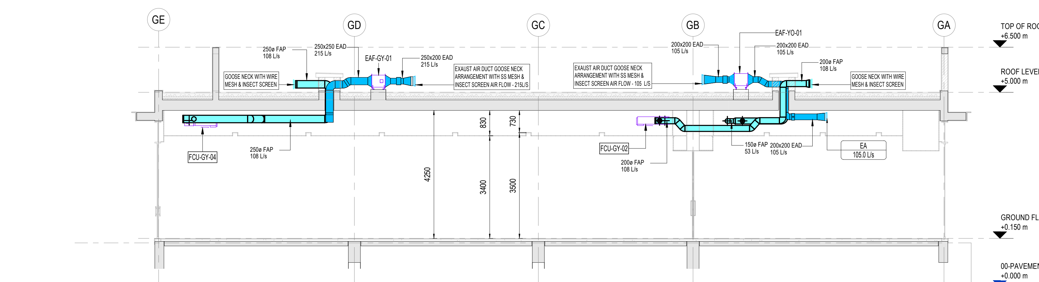
3 GYM&YOGA VENTILATION SECTION 01 1 : 75
