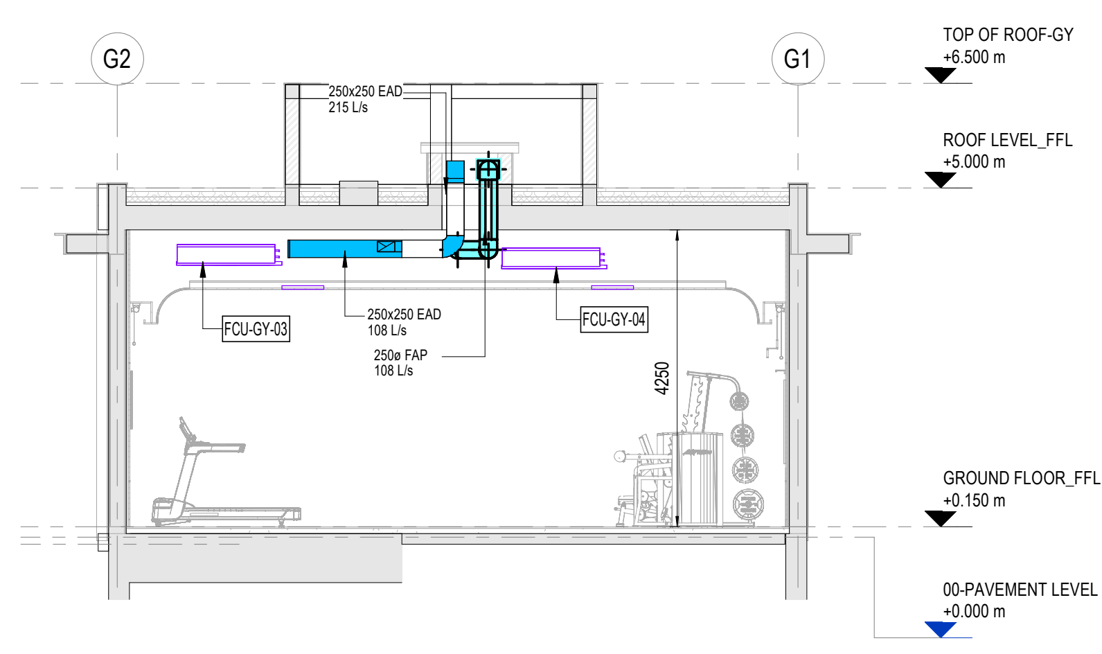
4 GYM&YOGA VENTILATION SECTION 02 1 : 75
