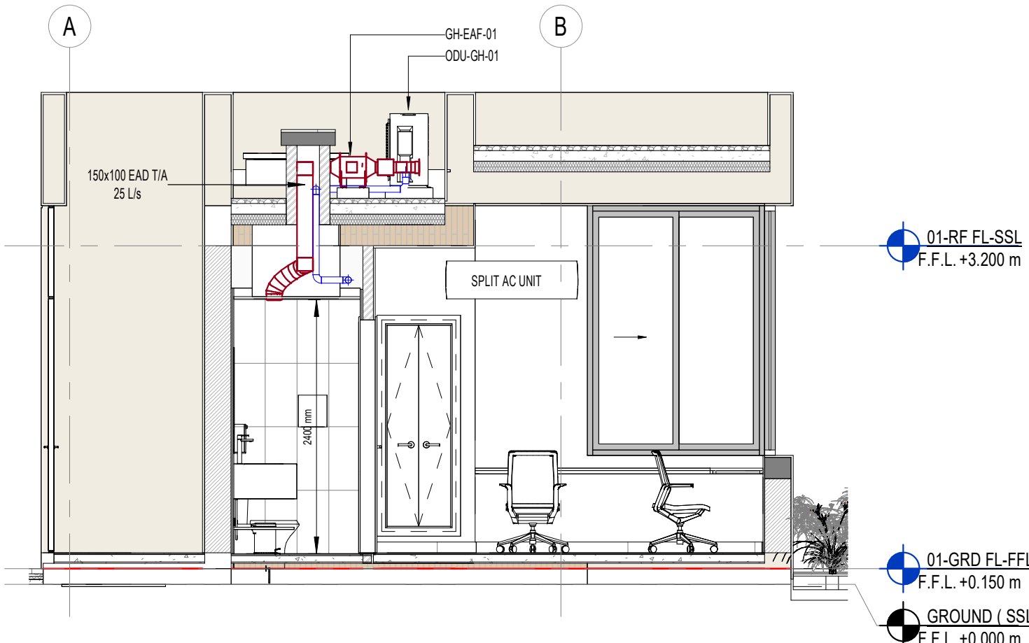
3 HVAC SECTION 1 1 : 50
