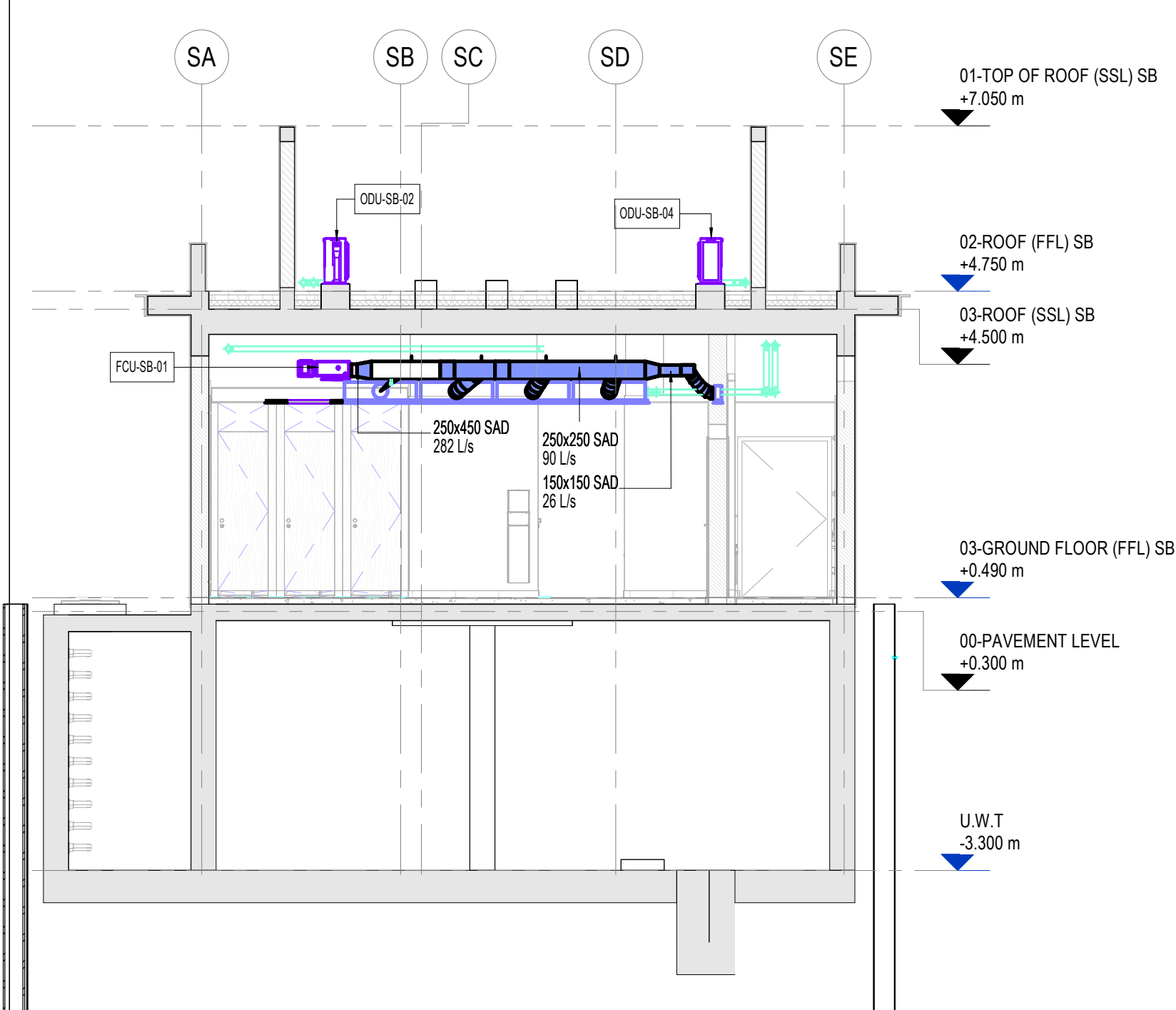
4 SERVICE BLOCK AC SECTION 01 1 : 75
