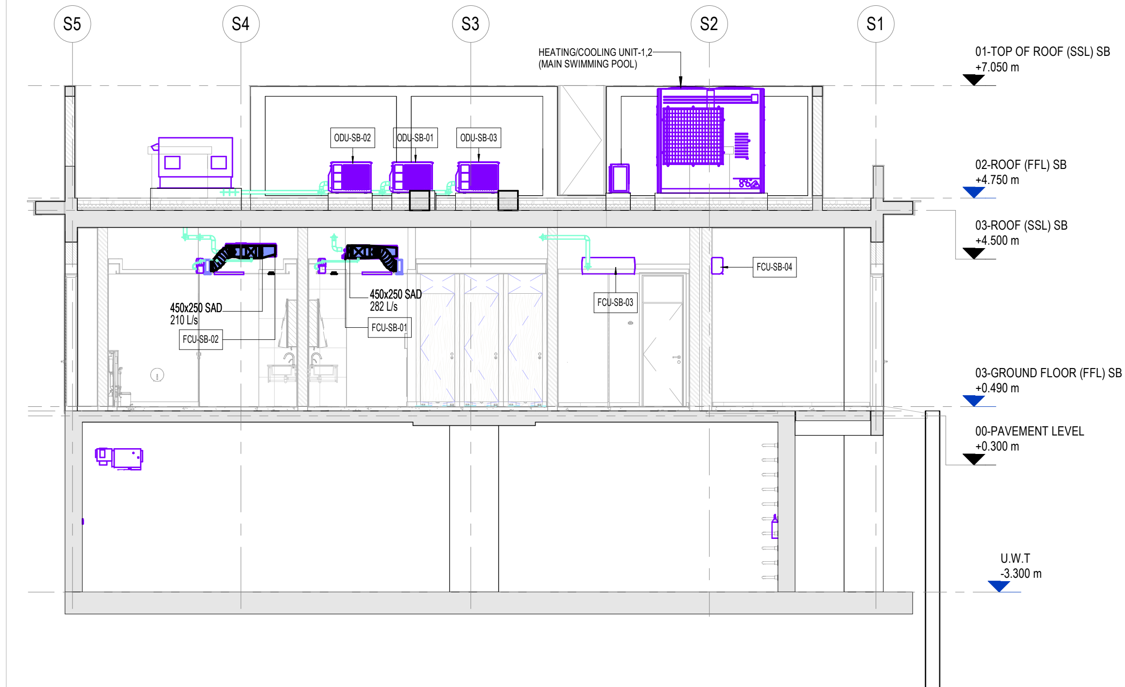
5 SERVICE BLOCK AC SECTION 02 1 : 75
