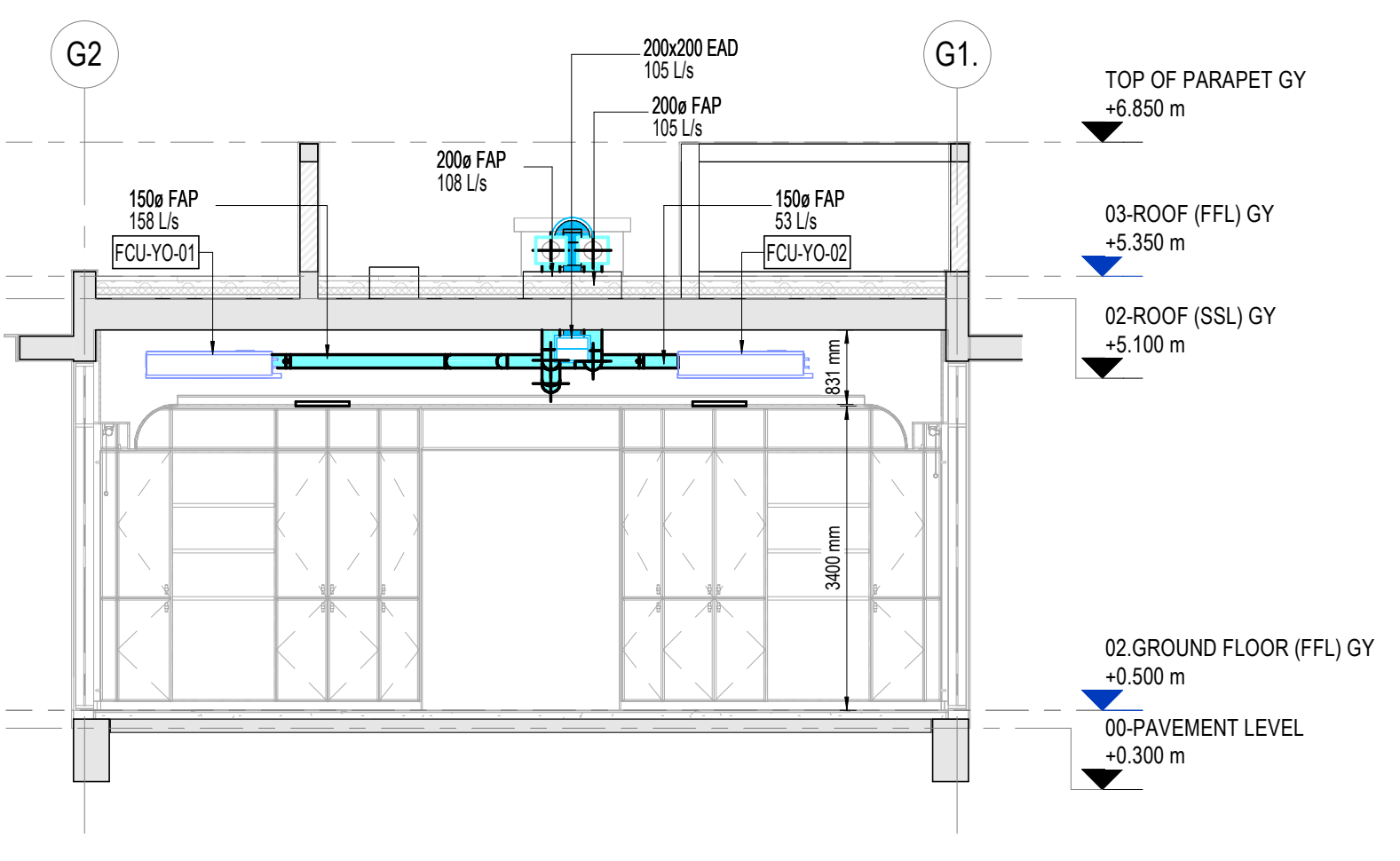
5 GYM&YOGA VENTILATION SECTION 03 1 : 75
