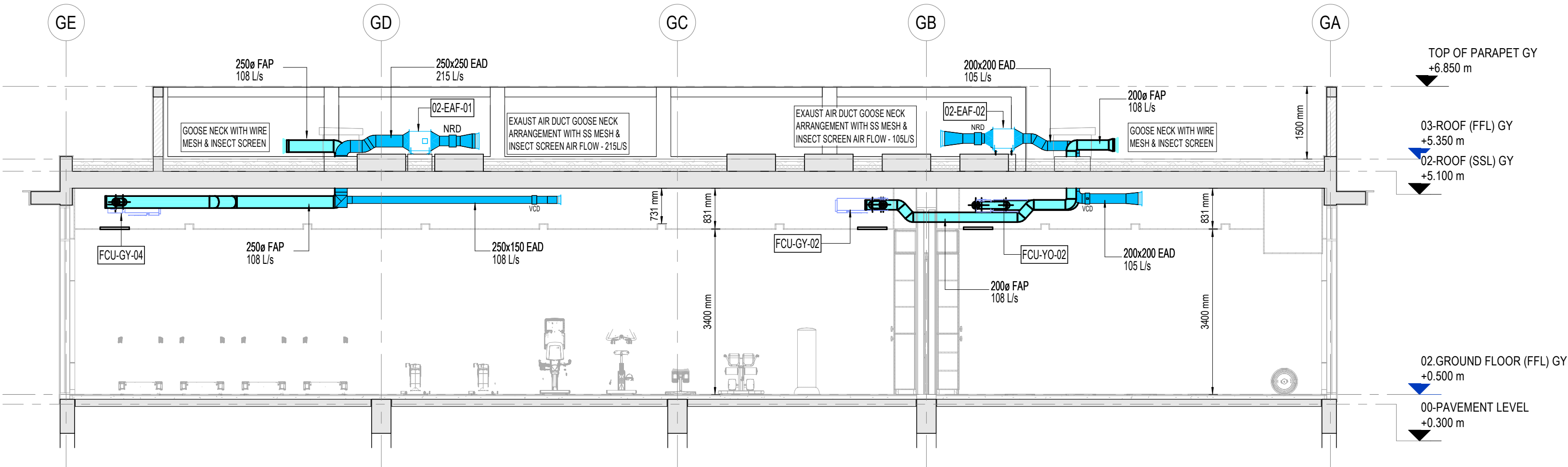
3 GYM&YOGA VENTILATION SECTION 02 1 : 75
