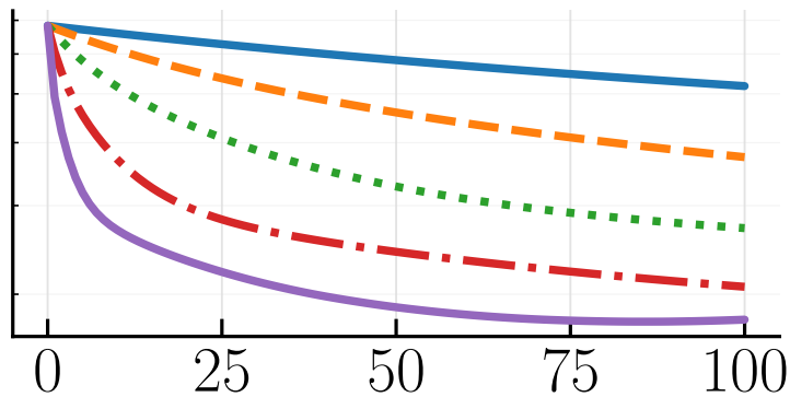
WFR
