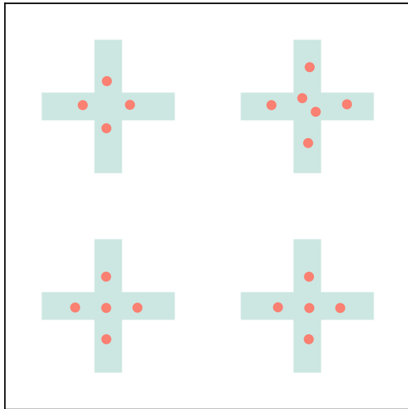
Ours
