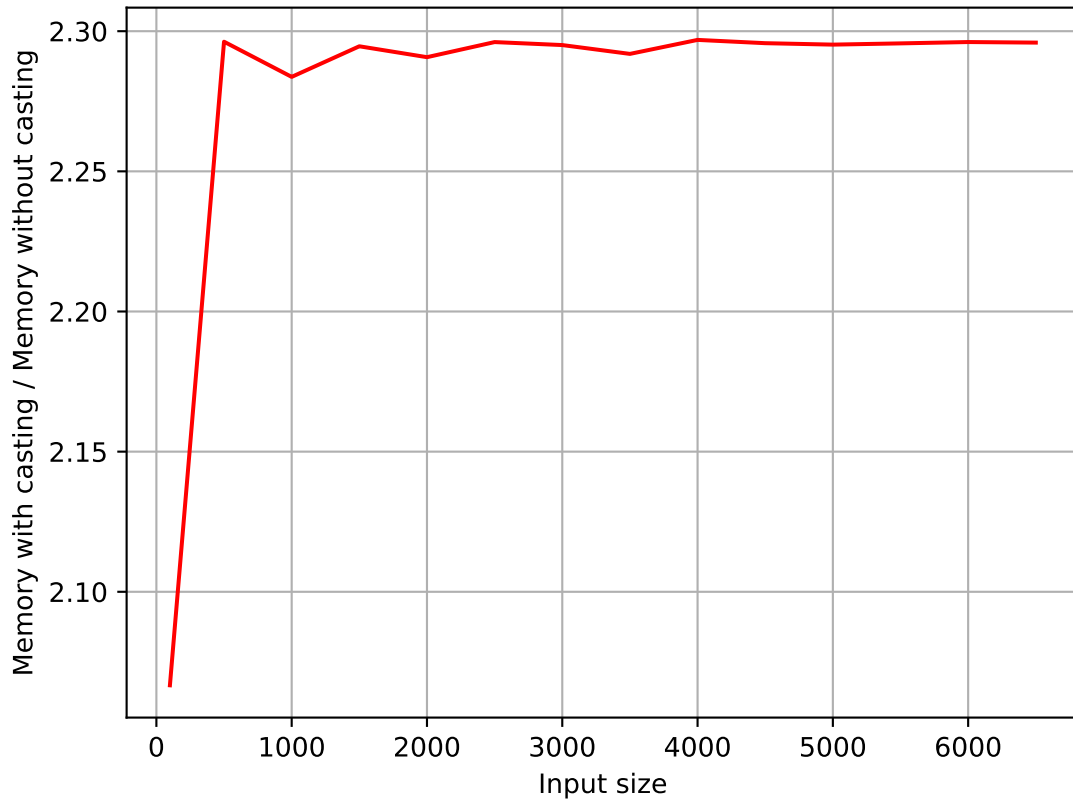
Llama3 8B
