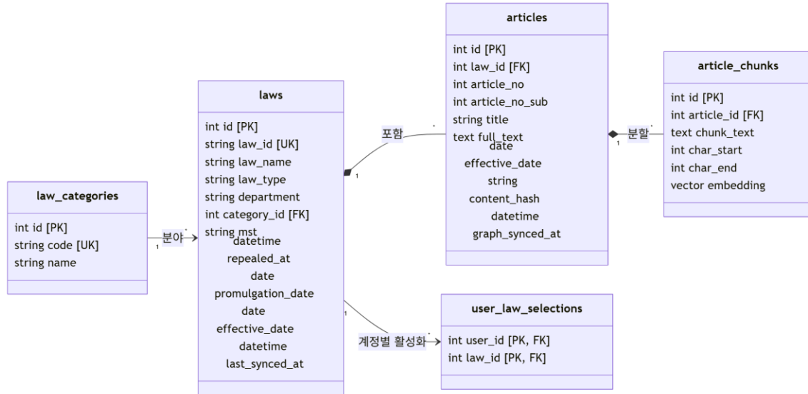
그림 3. 법령 검색 도메인 ERD
