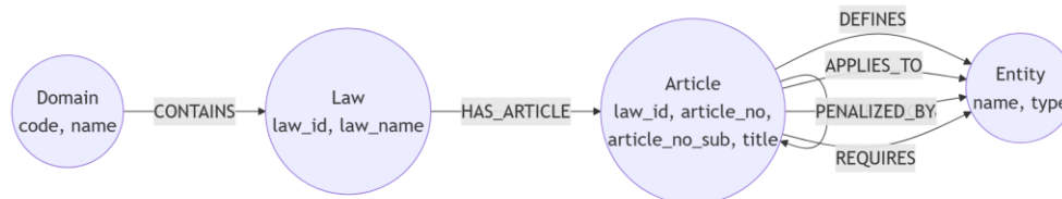
그림 4. 지식 그래프 도메인 ERD
