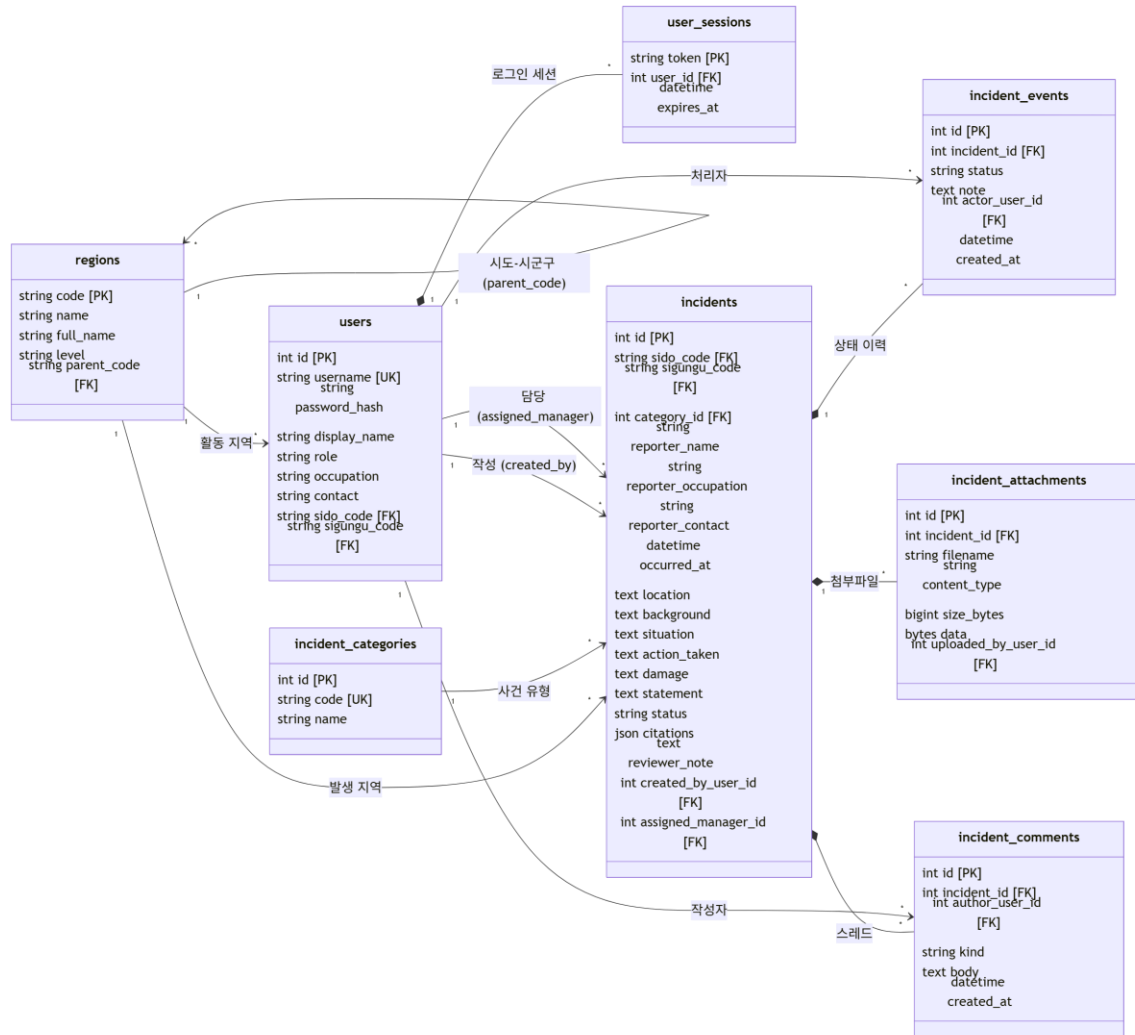
그림 5. 사건 관리 워크플로우 ERD
