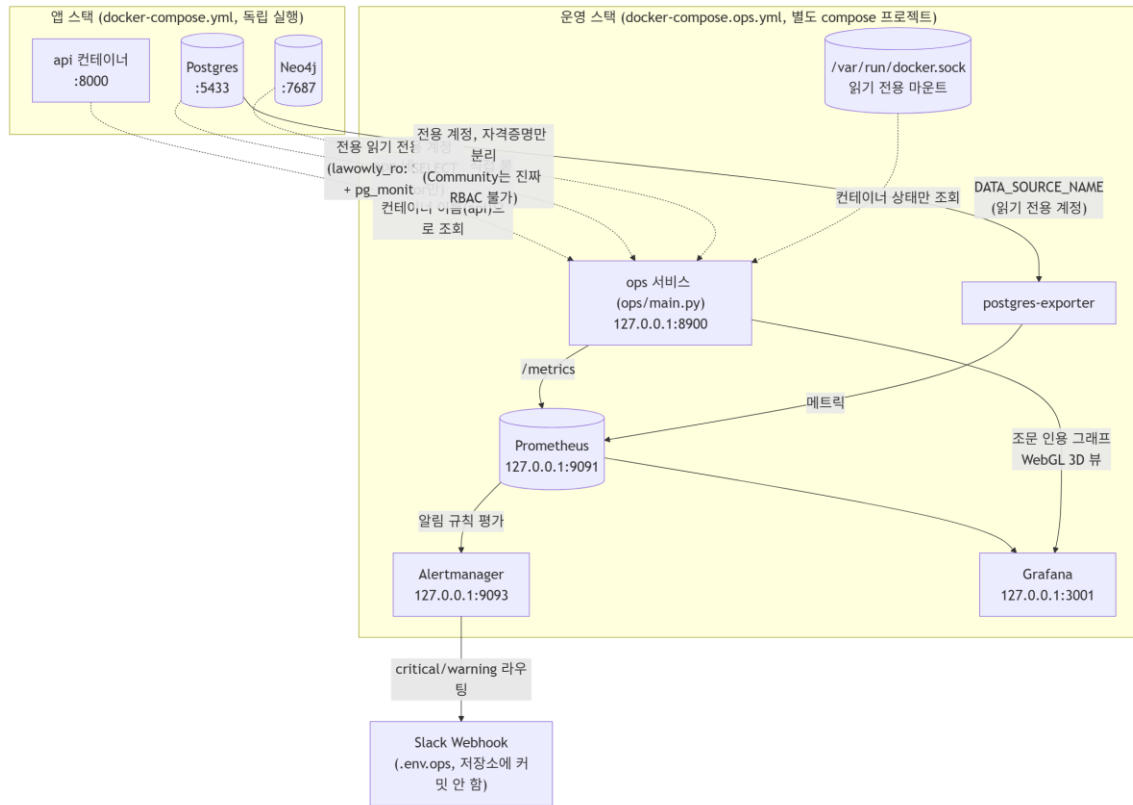
그림 6. 네트워크 포트 및 접근 정책
