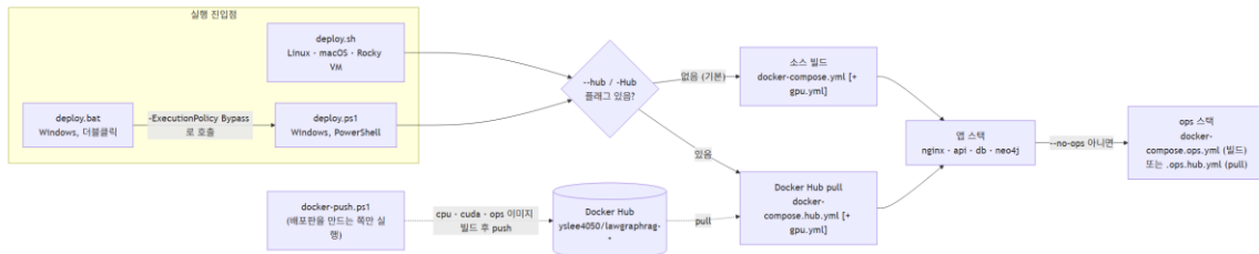
그림 1. 배포 및 실행 진입점 워크플로우
