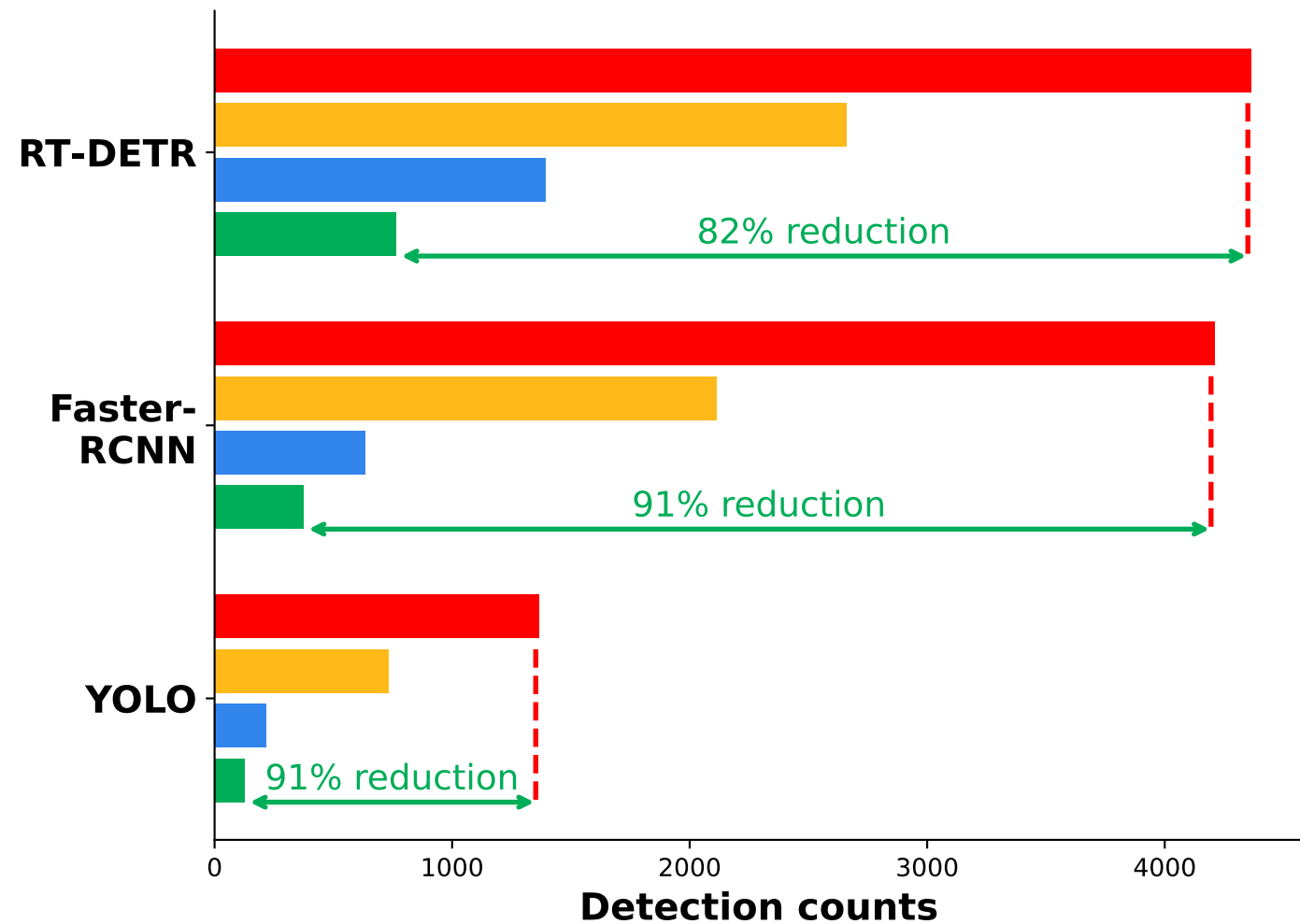
ID:BDD OoD:Near+Far
