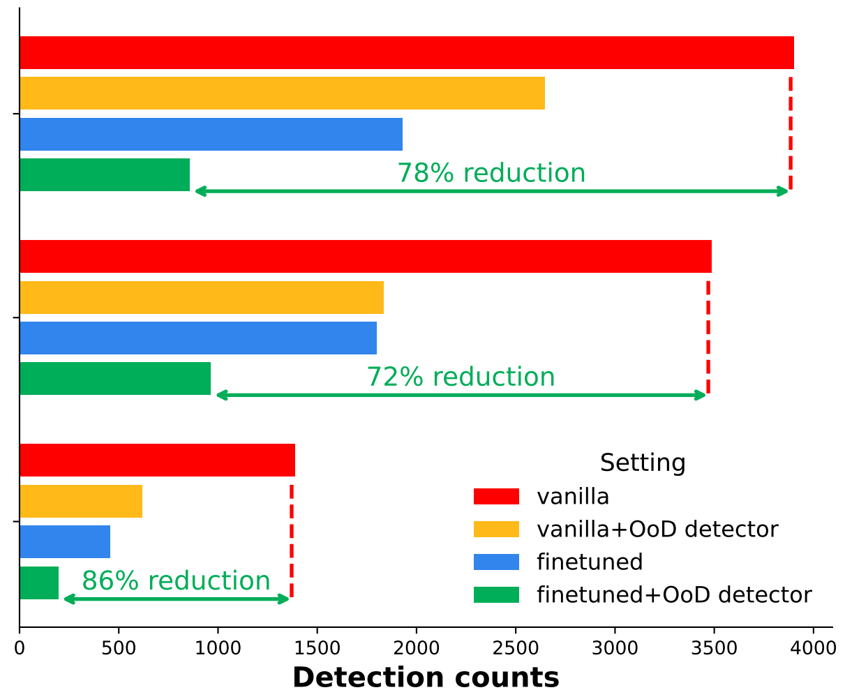
ID:VOC OoD:Near+Far
