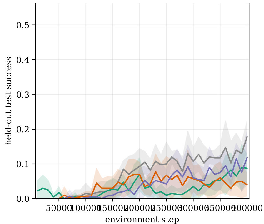
IQL
