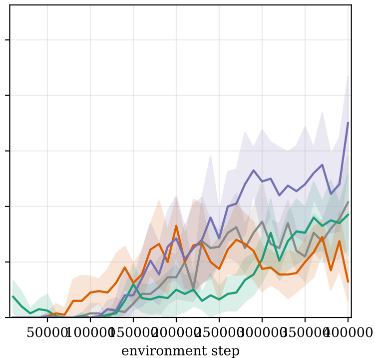
VDN
