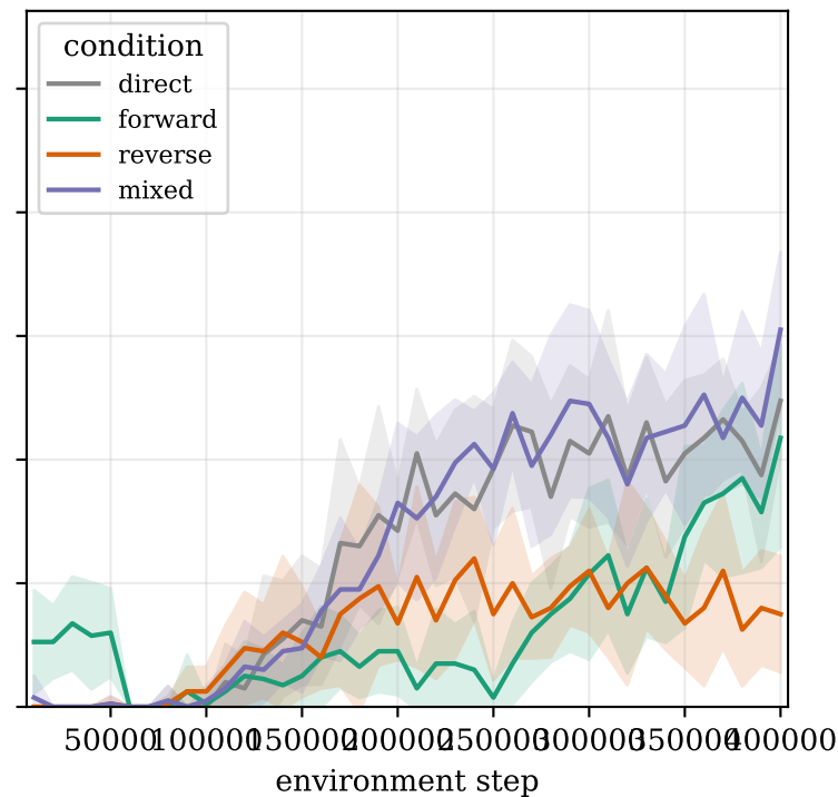
QMIX
