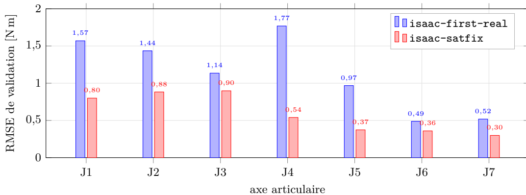
Figure 3 – Effet du filtrage de saturation (10) : RMSE de validation , avant et après. L'amélioration est présente sur les sept axes. Mesures antérieures à la partition à trois voies (16 juillet 2026), donc sur l'ensemble ayant servi à la sélection du point de contrôle : seul le signe de l'effet est exploitable, non son amplitude, et ces valeurs ne sont pas comparables à celles du reste de la section 6. La comparaison ne peut être refaite, le jeu de données antérieur au filtre n'existant plus.
