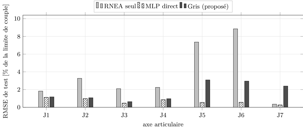
Figure 2 — Erreur de prédiction sur le jeu de test réservé (14 830 échantillons), rapportée à la limite de couple de chaque axe. La normalisation est nécessaire : en valeur absolue, les axes du poignet (limite 12 N m) sont illisibles à côté des axes porteurs (87 N m). Deux lectures s'imposent. D'une part le modèle analytique est au plus mal sur le poignet (axes 5 et 6), là où le modèle appris a donc le plus à apporter. D'autre part c'est précisément là que le modèle gris reste loin de la boîte noire, alors qu'il l'égale sur les axes 1 à 4 : l'écart global de tableau 1 est presque entièrement un écart de poignet. Les remarques de section 6.2 sur la partition des données s'appliquent aux trois séries.
