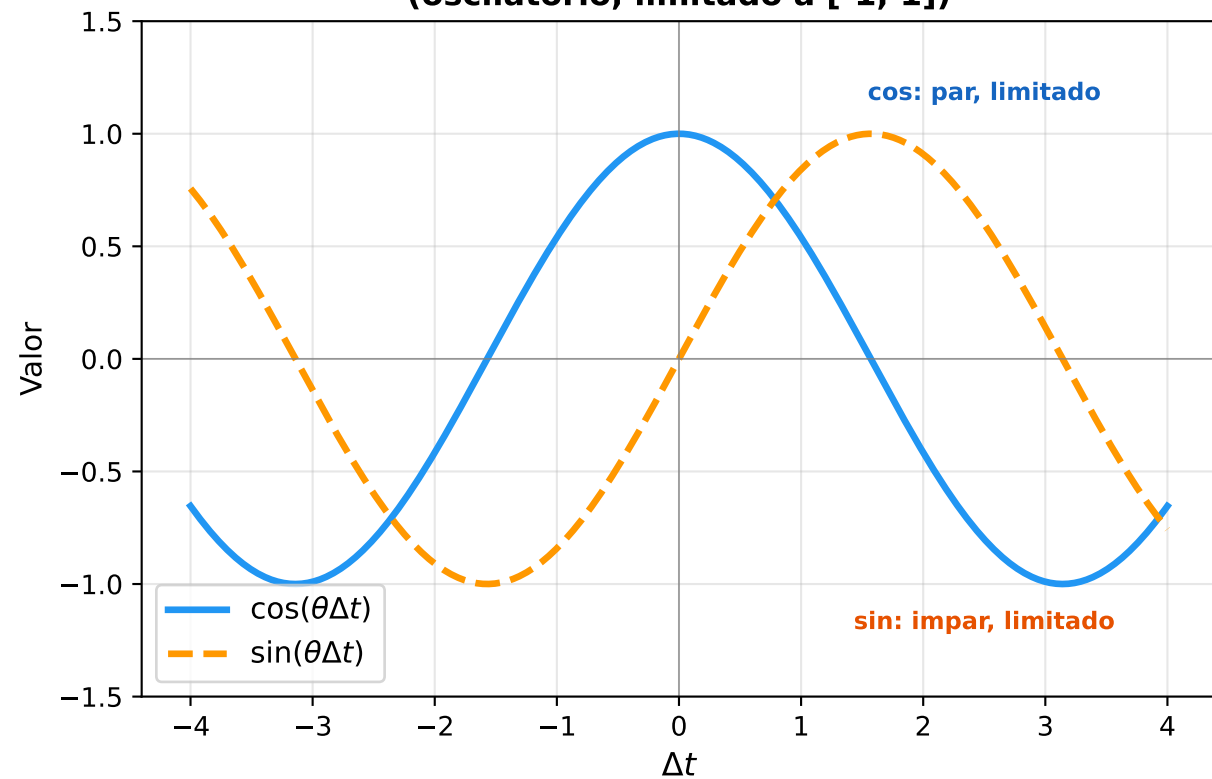
RoTHP: Kernel Trigonometrico (oscilatorio, limitado a [-1, 1] )
