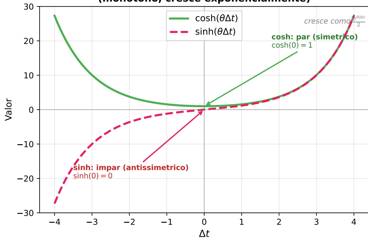
HoPE: Kernel Hiperbolico (puro) (monotono, cresce exponencialmente)
