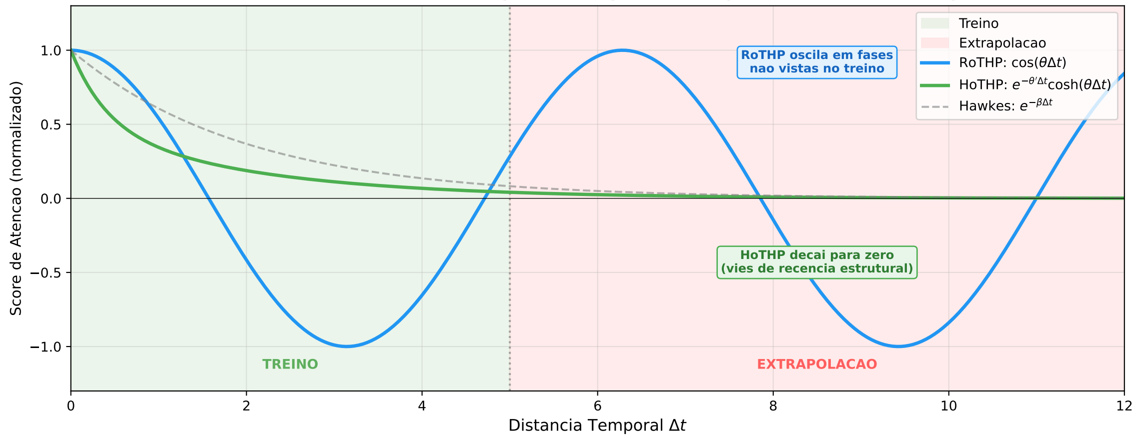
Kernel de Atencao: RoTHP (oscilatorio) vs HoTHP (decaimento monotono)
