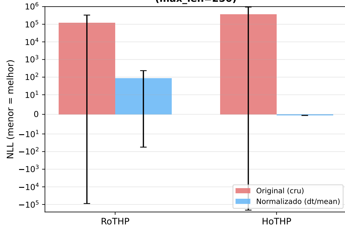
Retweet — 5x (max_len=250)
