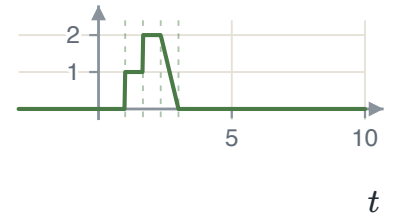
y(t) = x(3t - 5)
