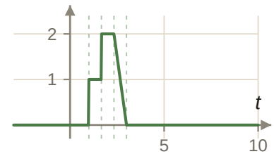
y(t) = x(3t - 5)
