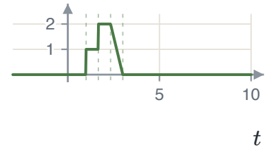
y(t) = x(3t - 5)
