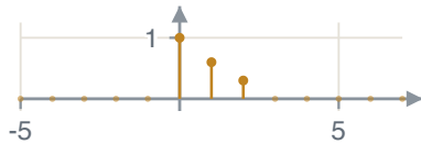
h[k]
