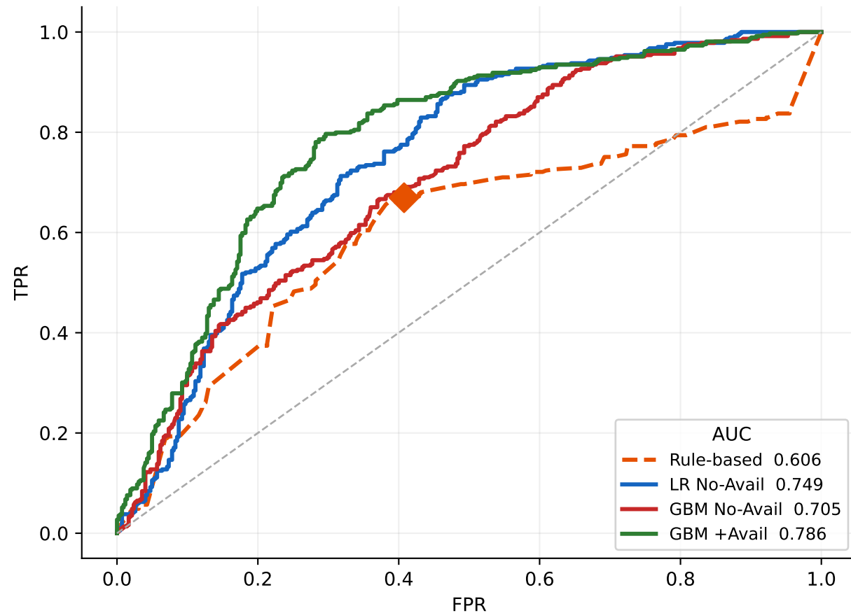
ROC Curve (OOF)
