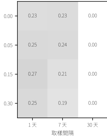
\tau_X = 30 天
