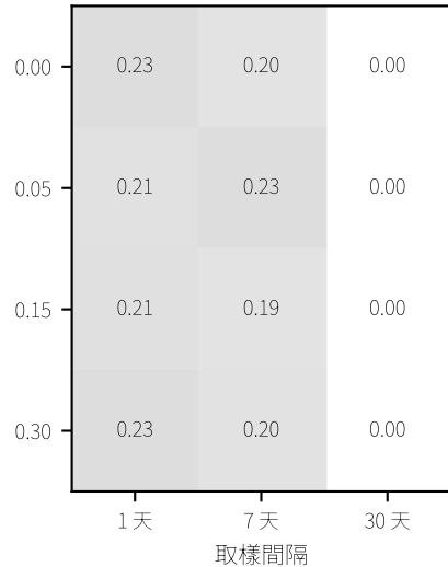
\tau_X = 90 天
