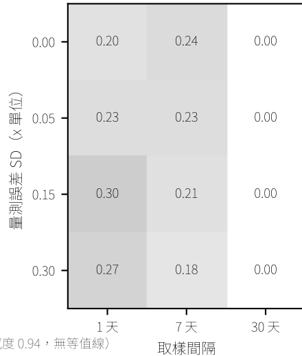
\tau_X = 14 天
