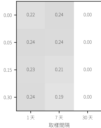
\tau_X = 60 天
