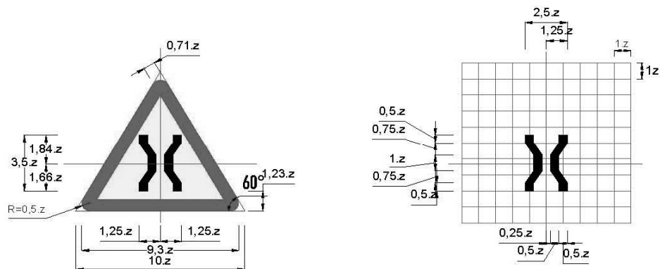
Biển số W.212: Cầu hẹp
