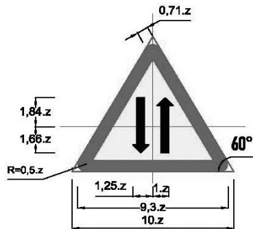
Biển số W.204: Đường hai chiều
