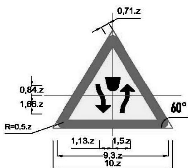
Biển số W.235: Đường đôi
