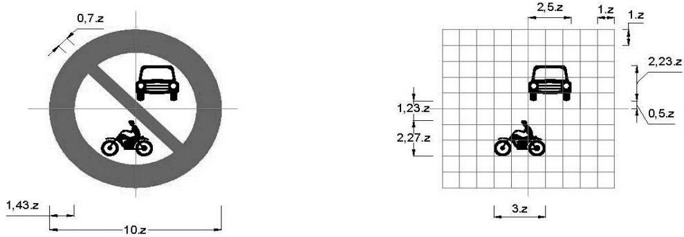
Biển số P.105: Cấm xe ô tô và xe mô tô
