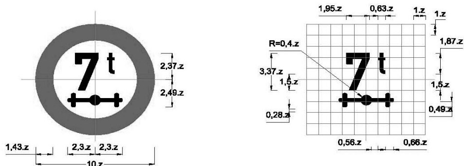
Biển số P.116: Hạn chế tải trọng trên trục xe
