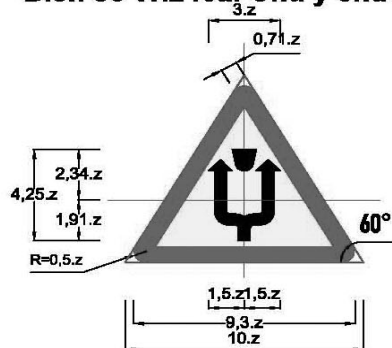
Biển số W.246a: Chú ý chướng ngại vật - Vòng tránh ra hai bên
