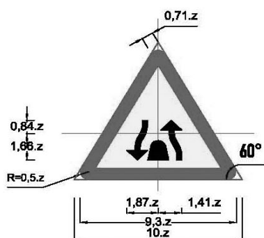
Biển số W.236: Hết đường đôi
