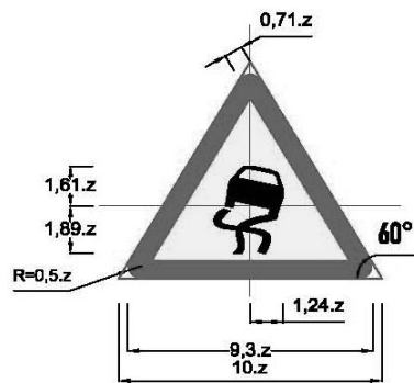
Biển số W.222a: Đường trơn
