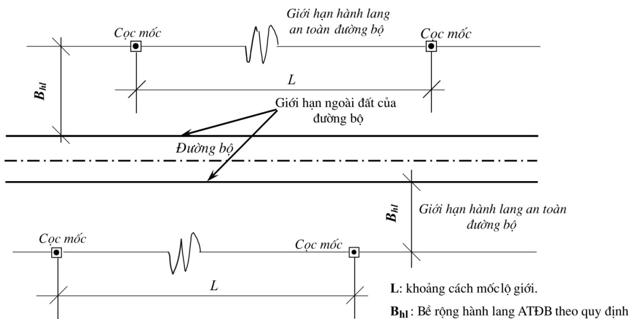
Hình I.4 - Cọc mốc lộ giới
