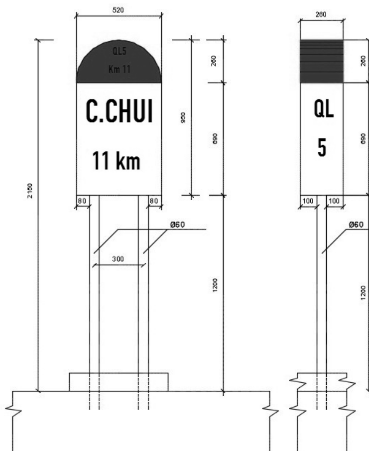
Hình I.1 - Cột kilômét dạng cột thấp
