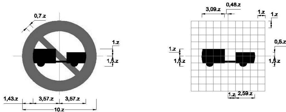
Biển số P.108: Cấm xe kéo rơ-moóc
