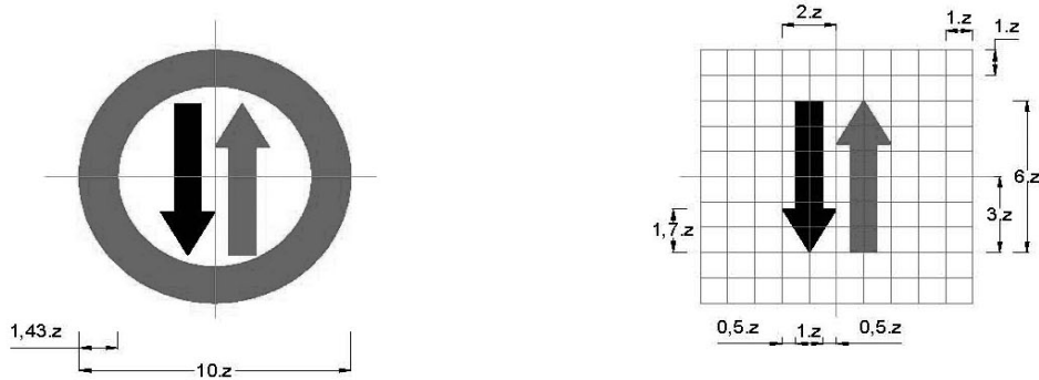
Biển số P.132: Nhường đường cho xe cơ giới đi ngược chiều qua đường hẹp
