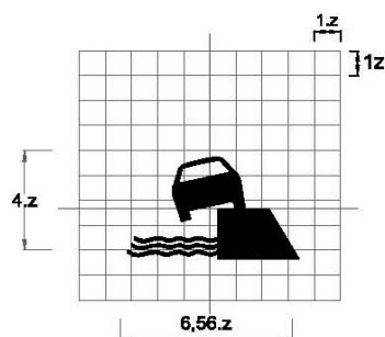
Biển số W.215c: Kè, vực sâu bên đường phía bên phải
