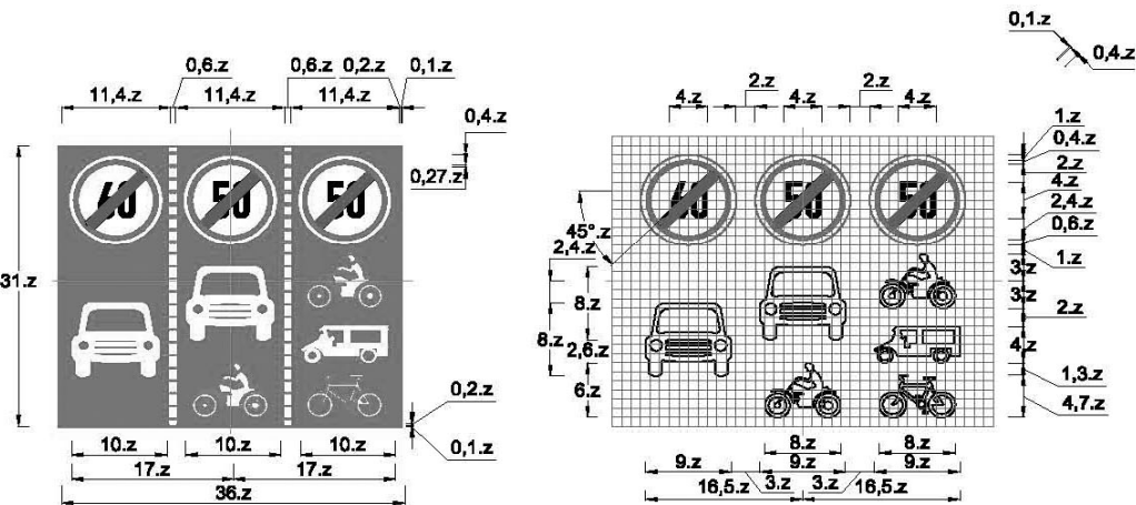
Biển số DP.127a
