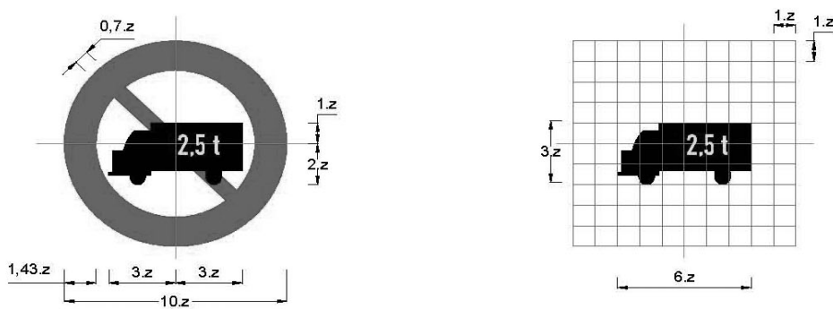
Biển số P.106b: Cấm xe ô tô tải
