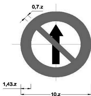
Biển số P.136: Cấm đi thẳng
