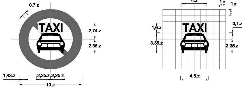
Biển số P.107b: Cấm xe ô tô taxi
