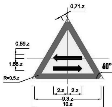
Biển số W.234: Giao nhau với đường hai chiều
