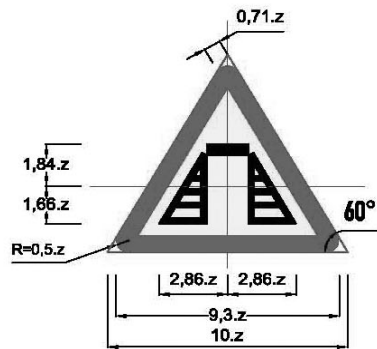
Biển số W.213: Cầu tạm
