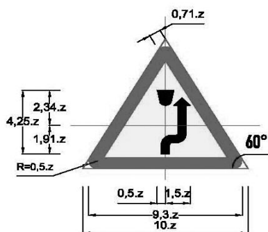
Biển số W.246c: Chú ý chướng ngại vật - Vòng tránh sang bên phải
