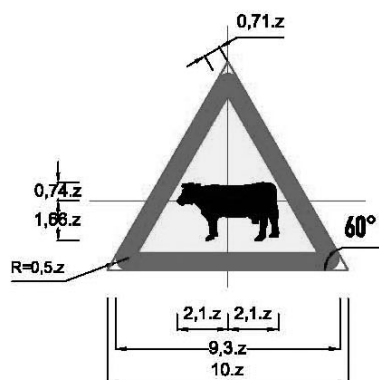
Biển số W.230: Gia súc
