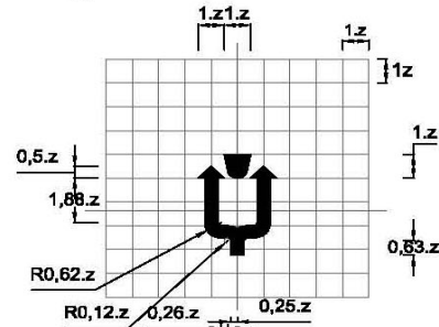
Biển số W.246a: Chú ý chướng ngại vật - Vòng tránh ra hai bên
