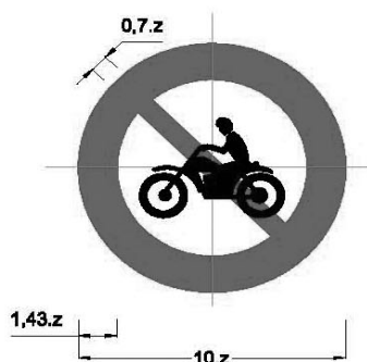
Biển số P.104: Cấm xe mô tô
