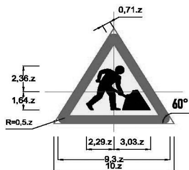
Biển số W.227: Công trường
