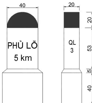
Hình I.1 - Cột kilômét dạng cột thấp
