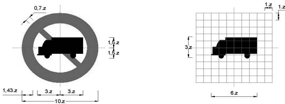
Biển số P.106a: Cấm xe ô tô tải
