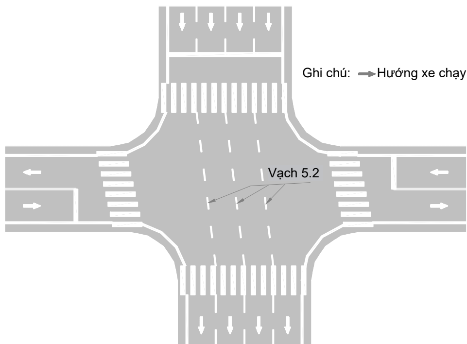
Hình G.41 - Minh họa bố trí vạch 5.2
