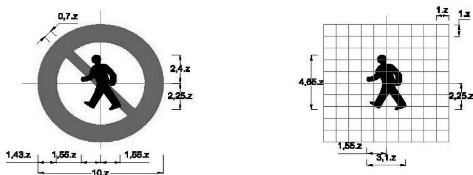
Biển số P.112: Cấm người đi bộ
