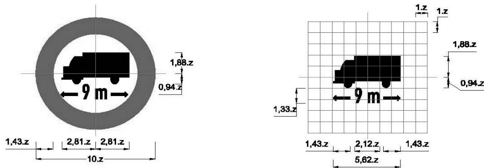
Biển số P.119: Hạn chế chiều dài xe
