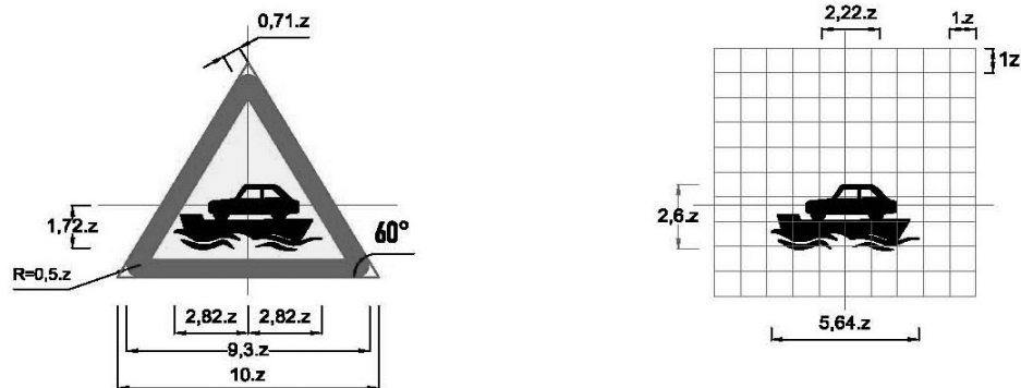
Biển số W.217: Bến phà
