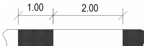
Hình G.68 - Chi tiết vạch 8.5
