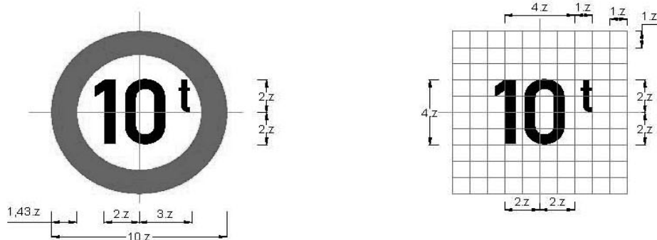
Biển số P.115: Hạn chế tải trọng toàn bộ xe
