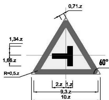
Biển số W.205c: Đường giao nhau
