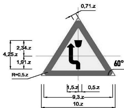
Biển số W.246b: Chú ý chướng ngại vật - Vòng tránh sang bên trái
