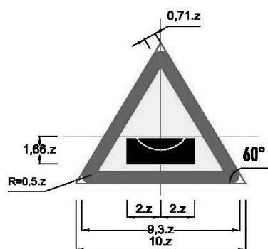
Biển số W.216a: Đường ngầm
