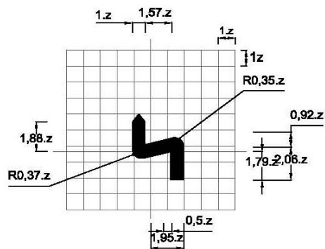
Biển số W.202a: Nhiều chỗ ngoặt nguy hiểm liên tiếp mà chỗ ngoặt đầu tiên hướng vòng bên trái
