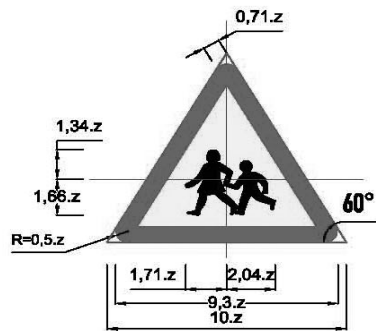
Biển số W.225: Trẻ em
