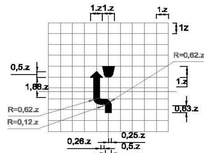
Biển số W.246b: Chú ý chướng ngại vật - Vòng tránh sang bên trái
