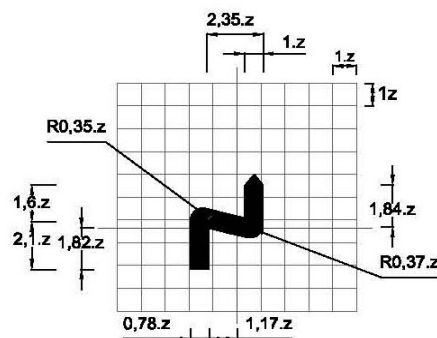
Biển số W.202b: Nhiều chỗ ngoặt nguy hiểm liên tiếp mà chỗ ngoặt đầu tiên hướng vòng bên phải
