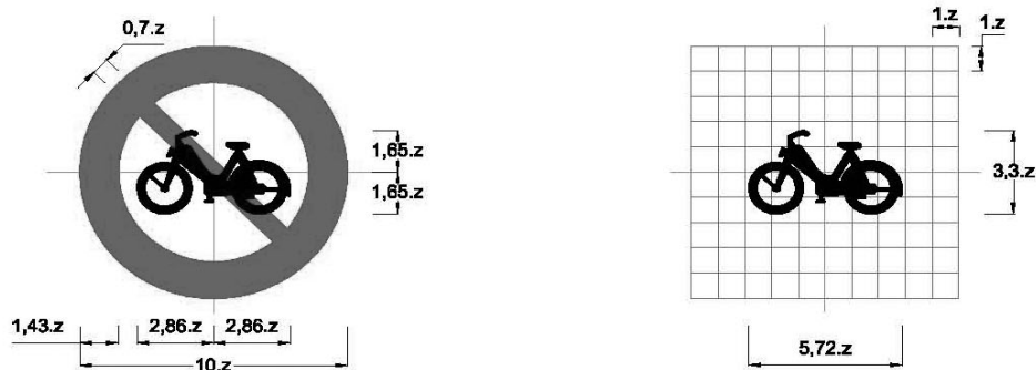
Biển số P.111a: Cấm xe gắn máy
