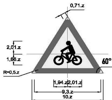
Biển số W.226: Đường người đi xe đạp cắt ngang
