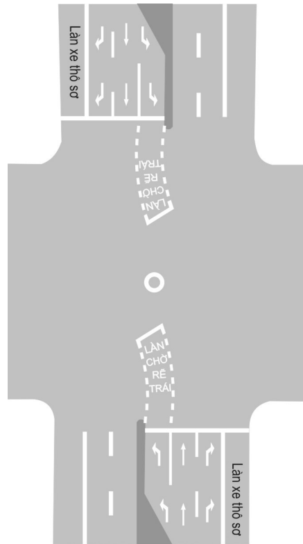
Hình G.42 - Minh họa bố trí vạch 5.3
