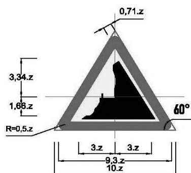
Biển số W.223b: Vách núi nguy hiểm
