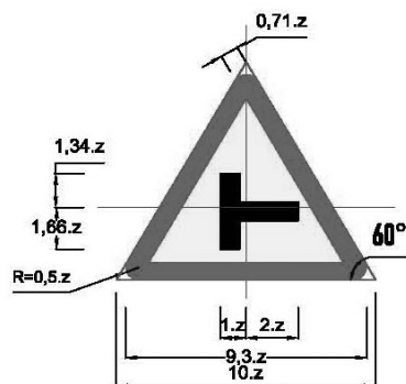
Biển số W.205b: Đường giao nhau
