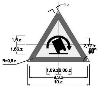
Biển số W.201c: Chỗ ngoặt nguy hiểm có nguy cơ lật xe bên phải khi đường cong vòng sang phải
