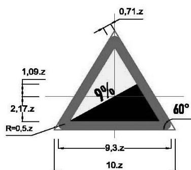
Biển số W.220: Dốc lên nguy hiểm
