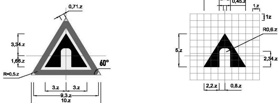
Biển số W.218: Cửa chui
