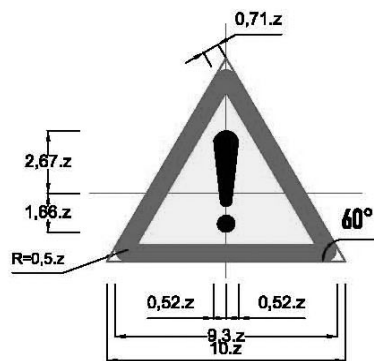
Biển số W.233: Nguy hiểm khác
