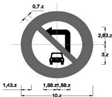
Biển số P.103c: Cấm xe ô tô rẽ trái
