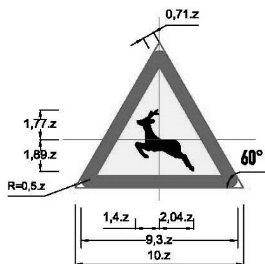
Biển số W.231: Thú rừng vượt qua đường
