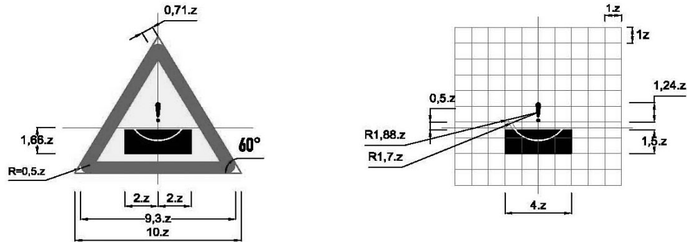
Biển số W.216b: Đường ngầm có nguy cơ lũ quét
