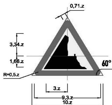
Biển số W.223a: Vách núi nguy hiểm
