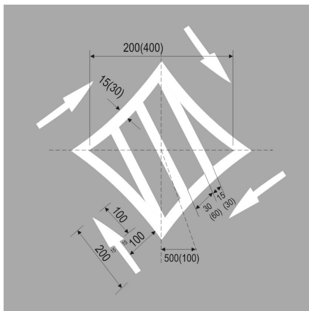
Hình G.37 - Vạch vành khuyên - Mẫu 2
