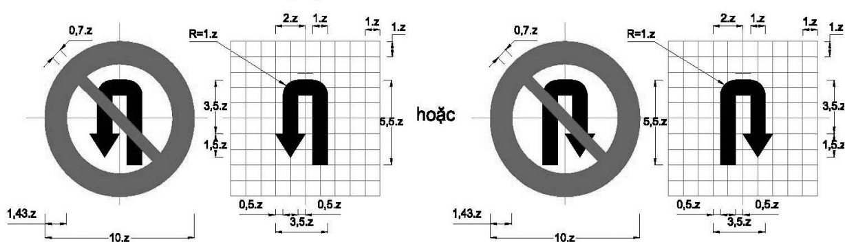
Biển số P.124a: Cấm quay đầu xe
