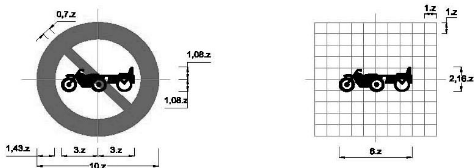
Biển số P.111c: Cấm xe ba bánh loại có động cơ
