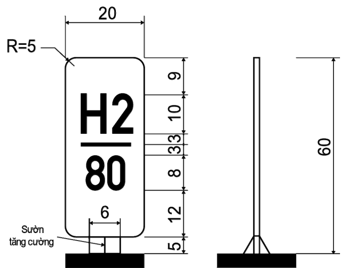
b) Cọc H dạng tấm
