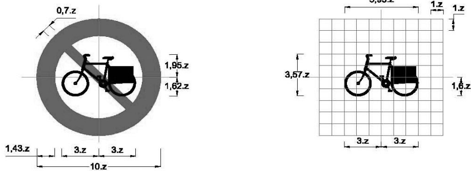
Biển số P.110b: Cấm xe đạp thồ
