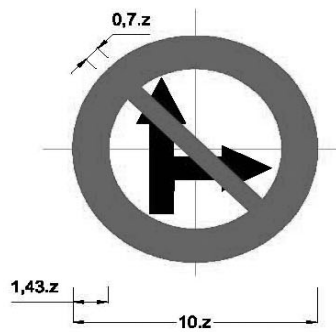
Biển số P.139: Cấm đi thẳng, rẽ phải
