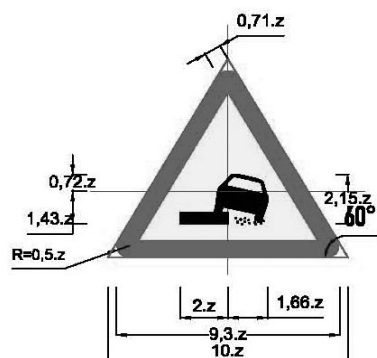
Biển số W.222b: Lề đường nguy hiểm
