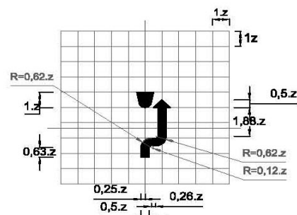
Biển số W.246c: Chú ý chướng ngại vật - Vòng tránh sang bên phải
