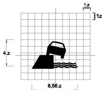
Biển số W.215b: Kè, vực sâu bên đường phía bên trái
