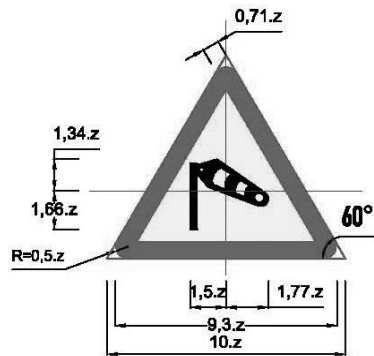
Biển số W.232: Gió ngang
