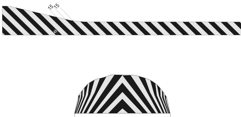
Hình G.64 - Sử dụng vạch 8.1 trên đảo phân làn tại trạm thu phí - Mẫu 2
