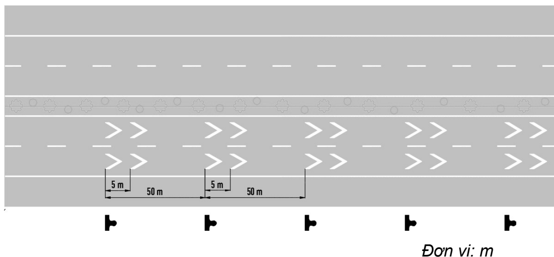
Hình G.57 - Bố trí vạch xác định khoảng cách xe trên đường
