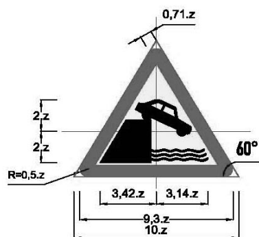
Biển số W.215a: Kè, vực sâu phía trước
