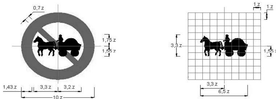
Biển số P.114: Cấm xe vật nuôi kéo
