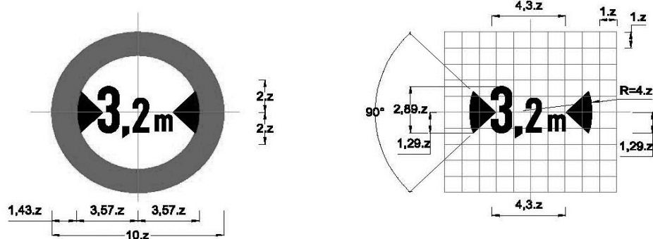
Biển số P.118: Hạn chế chiều ngang xe
