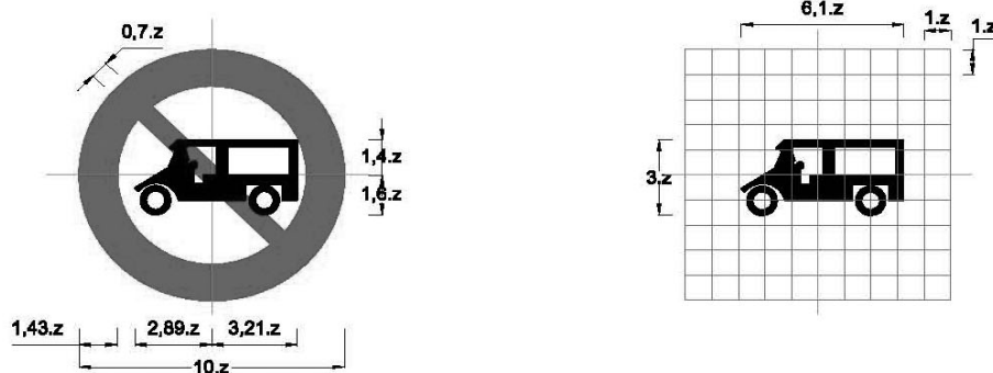
Biển số P.111b: Cấm xe ba bánh loại có động cơ
