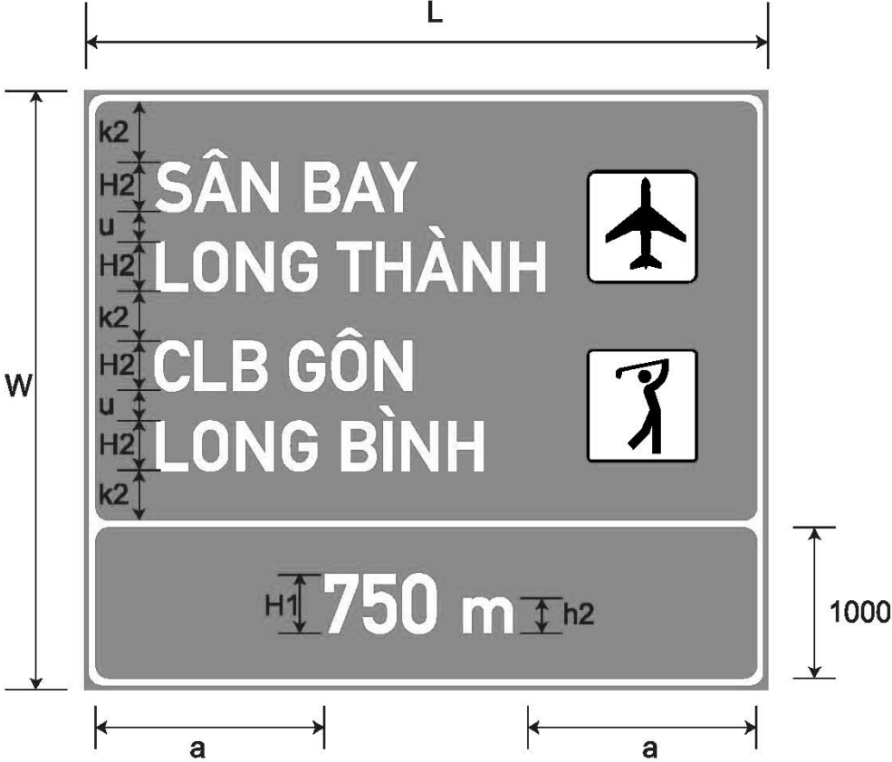
a) Biển số IE.461a:
