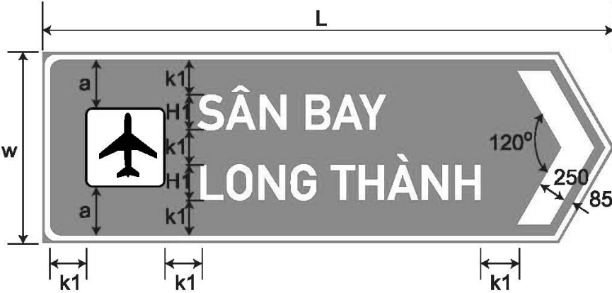
d) Biển số IE.461d:
