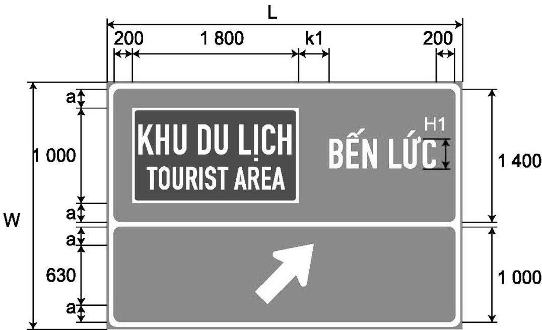
b) Biển số IE.459b:
