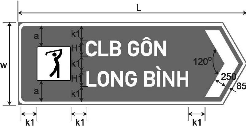
d) Biển số IE.461d:
