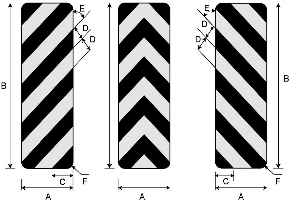
Biển số IE.468a
