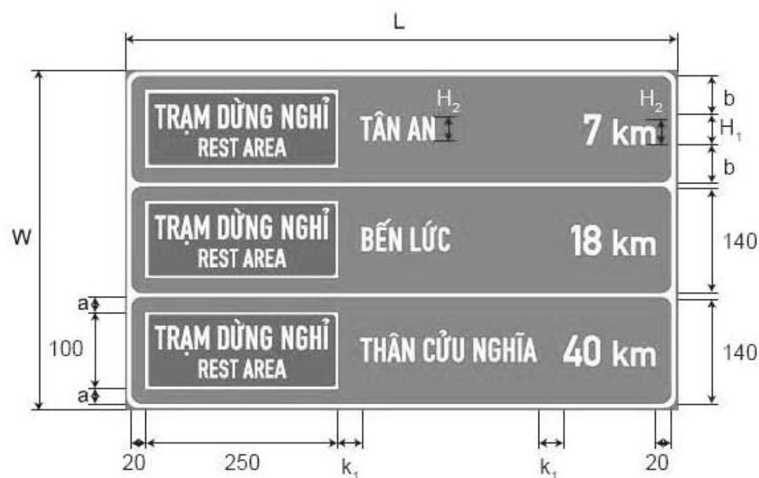
P.10 Biển chỉ dẫn khoảng cách để các trạm dừng nghỉ tiếp theo a) Biển số IE.458:
