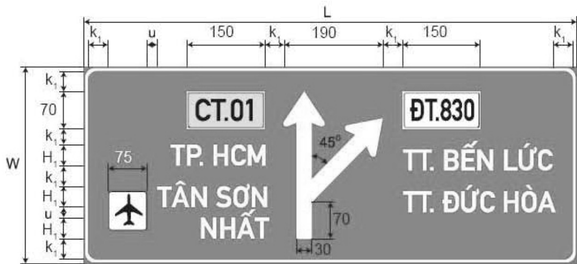
P.18 Biển chỉ dẫn sơ đồ lối ra Biển số IE.466
