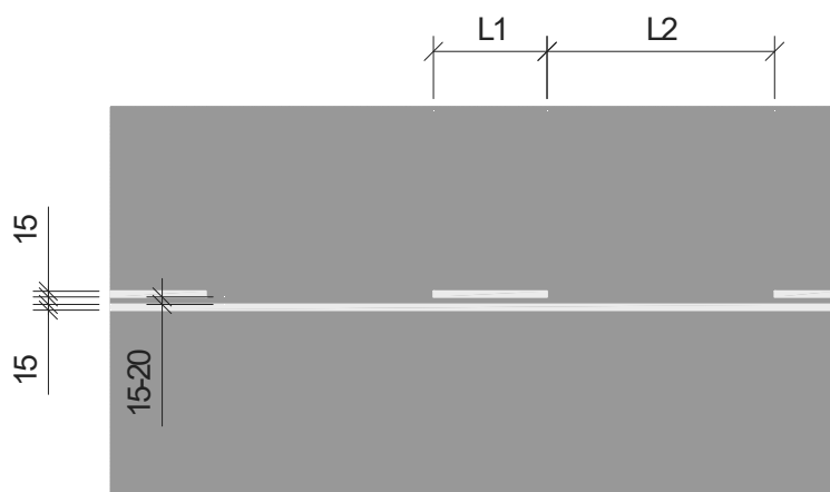
Hình G.4 - Vạch 1.4
