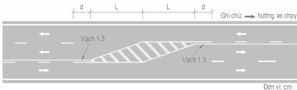
Hình G.8 - Bố trí vạch sơn phân chia hai chiều xe chạy cho đường có 3 làn xe trong khu vực số làn trên một hướng thay đổi từ một làn sang hai làn
