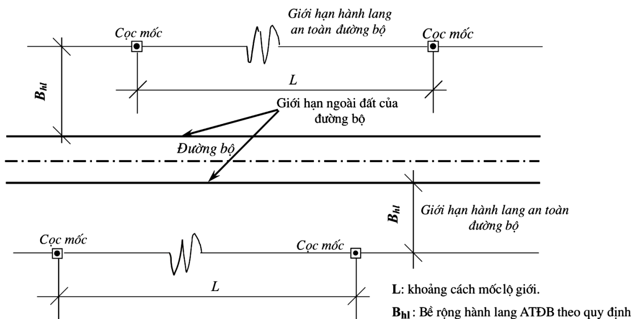
Hình I.5 - Mặt bằng bố trí cọc lộ giới
