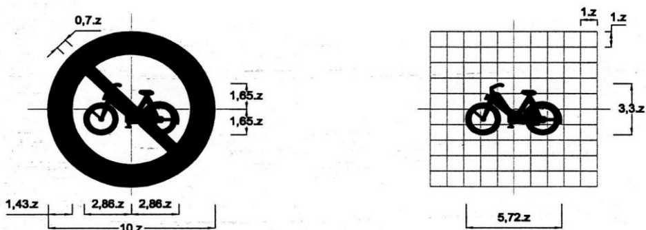
Biển số P.111a: Cấm xe gắn máy
