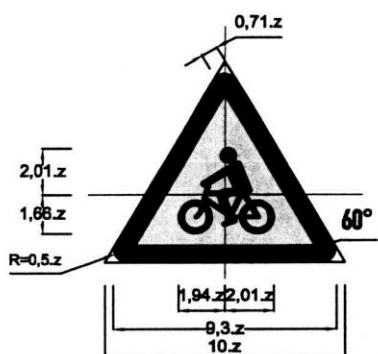
Biển số W.226: Đường người đi xe đạp cắt ngang
