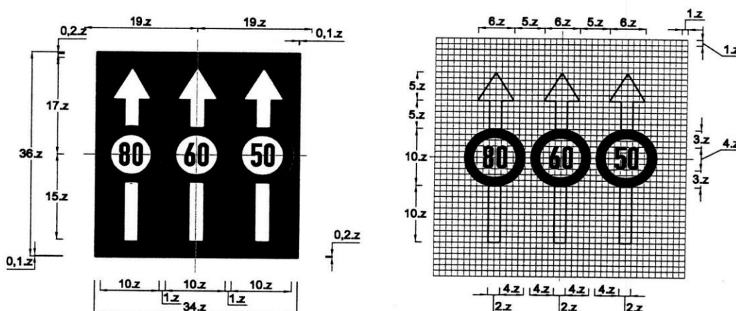
Biển số P.127b: Biển gộp tốc độ tối đa cho phép theo làn đường đặt bên đường hoặc trên cột cần vịn
