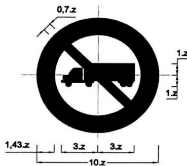
Biển số P.108a: Cấm xe sơ-mi-rơ-móc
