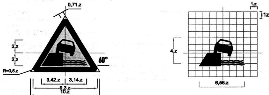
Biển số W.215b: Kè, vực sâu bên đường phía bên trái
