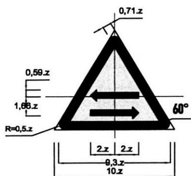
Biển số W.234: Giao nhau với đường hai chiều
