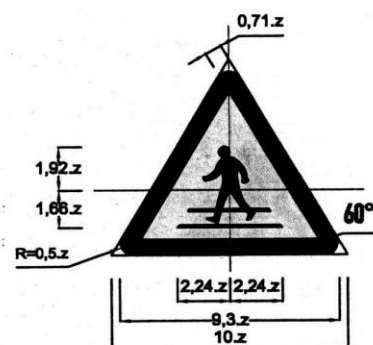
Biển số W.224: Đường người đi bộ cắt ngang
