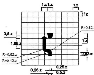
Biển số W.246b: Chú ý chướng ngại vật - Vòng tránh sang bên trái
