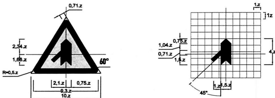
Biển số W.207f: Giao nhau với đường không ưu tiên
