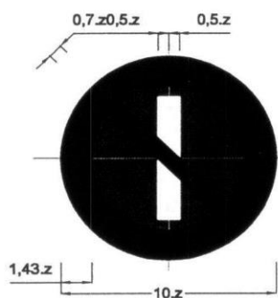
Biển số P.131b: Cấm đỗ xe vào ngày lẻ
