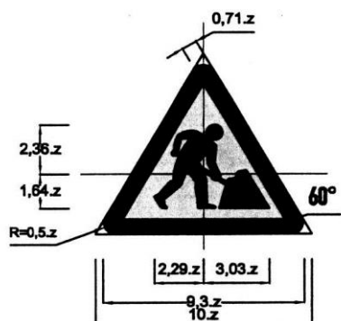
Biển số W.227: Công trường
