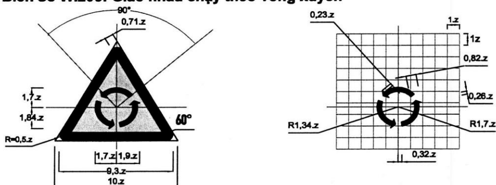
Biển số W.206: Giao nhau chạy theo vòng xuyến
