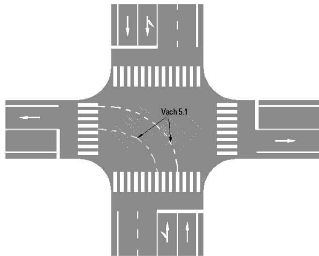
Hình G.40 - Minh họa bố trí vạch 5.1
