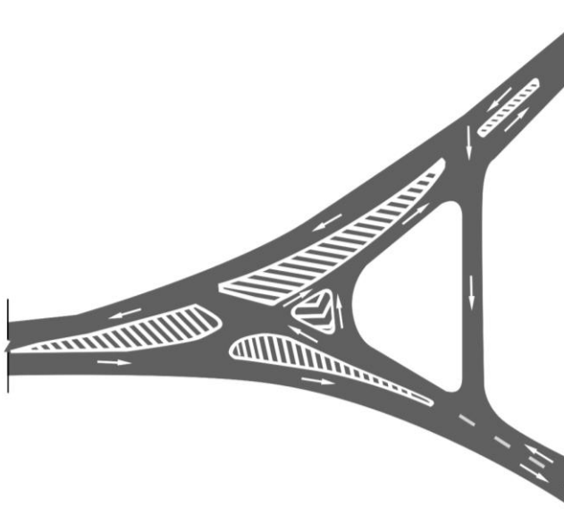
Hình G.32 - Bố trí vạch kênh hóa dòng xe ở ngã ba phức tạp - Mẫu 3
