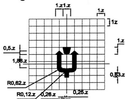
Biển số W.246a: Chú ý chướng ngại vật - Vòng tránh ra hai bên
