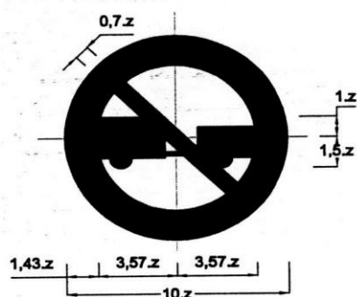
Biển số P.108: Cấm xe kéo rơ-moóc
