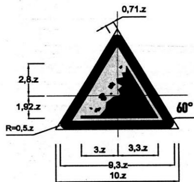
Biển số W.228b: Đá lở
