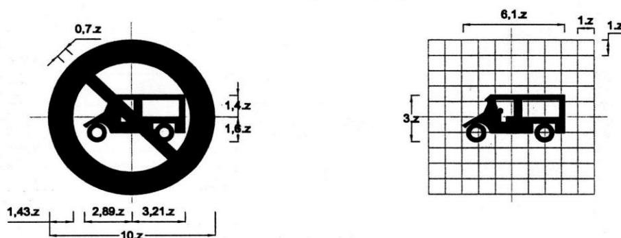
Biển số P.111b: Cấm xe ba bánh loại có động cơ
