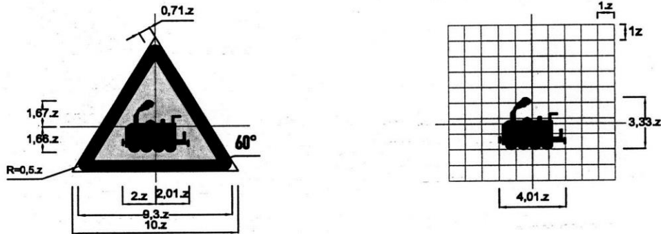
Biển số W.211a: Giao nhau với đường sắt không có rào chắn
