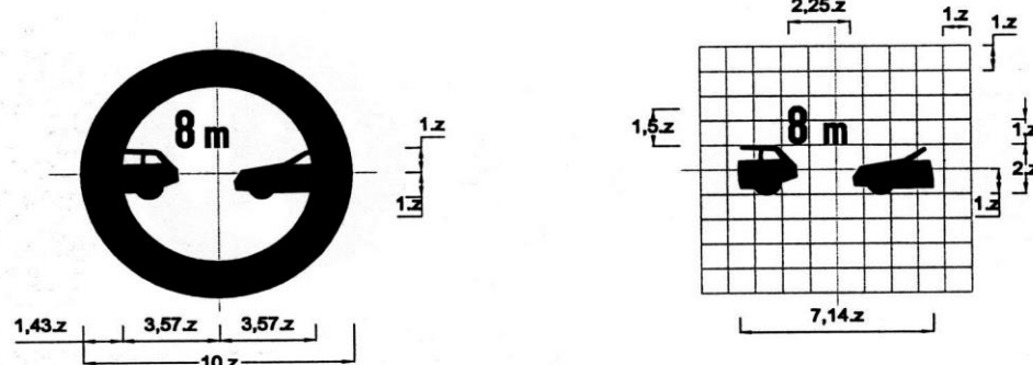
Biển số P.121: Cự ly tối thiểu giữa hai xe
