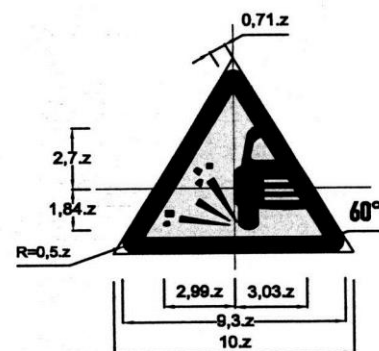
Biển số W.228c: Sỏi đá bắn lên
