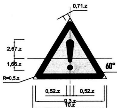
Biển số W.233: Nguy hiểm khác
