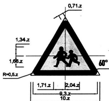
Biển số W.225: Trẻ em
