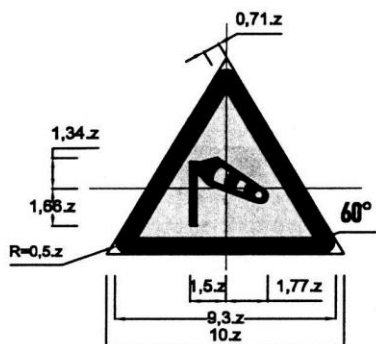
Biển số W.232: Gió ngang
