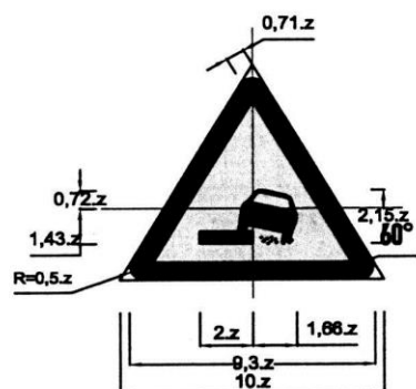
Biển số W.222b: Lề đường nguy hiểm
