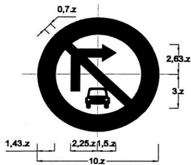
Biển số P.103b: Cấm xe ô tô rẽ phải
