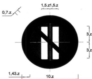
Biển số P.131c: Cấm đỗ xe vào ngày chẵn
