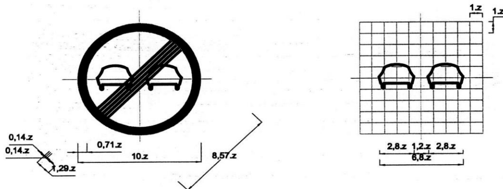
Biển DP.133: Hết cấm vượt
