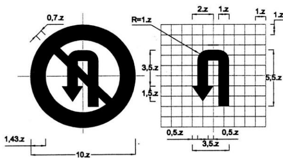
Biển số P.124a: Cấm quay đầu xe
