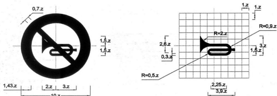
Biển số P.128: Cấm sử dụng còi
