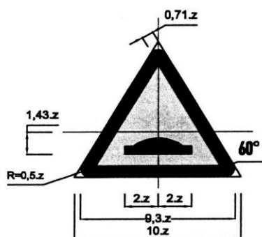
Biển số W.221b: Đường có gờ giảm tốc
