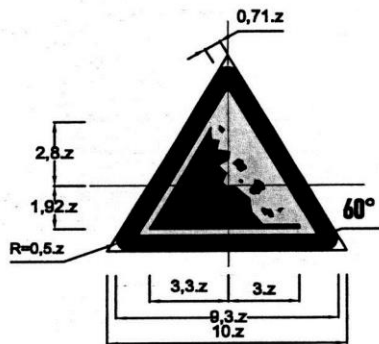
Biển số W.228a: Đá lở
