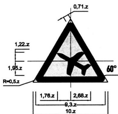
Biển số W.229: Dải máy bay lên xuống
