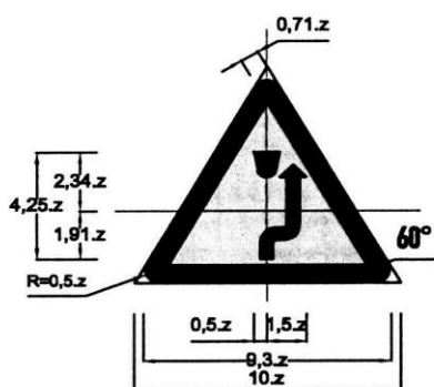
Biển số W.246c: Chú ý chướng ngại vật - Vòng tránh sang bên phải
