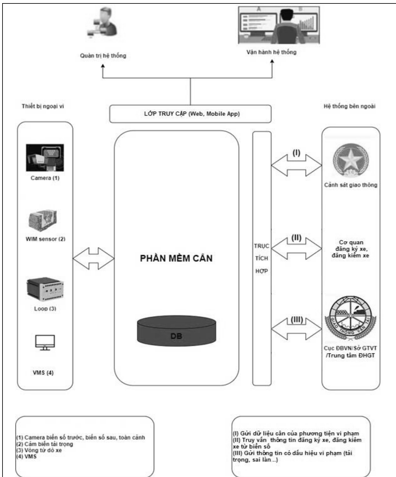
Hình A-1: Sơ đồ minh họa mô hình chung công trình KSTTX
