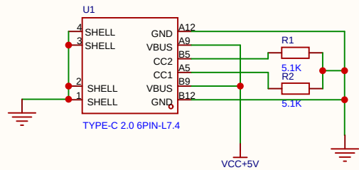
电源电路
