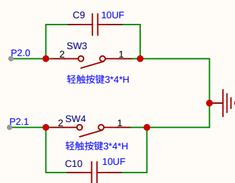
按键检测电路
