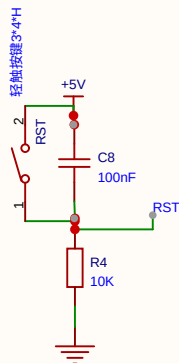
复位电路
