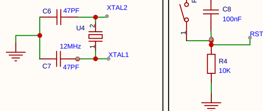
晶振电路
