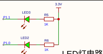
LED灯电路
