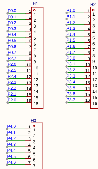
单片机引脚引出
