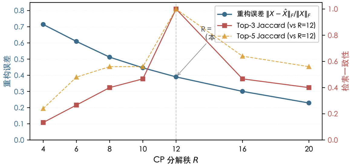
Fig. 7 CP 分解秩 R 对重构误差与检索一致性的影响
