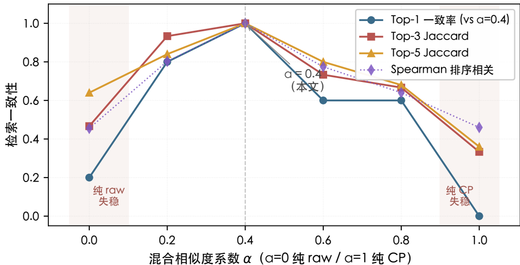
Fig. 8 混合相似度 \alpha 对检索一致性的影响 ( R = 12 固定)
