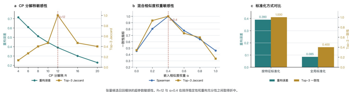
图 5 张量召回模块超参数敏感性 Fig. 5 Hyperparameter sensitivity of the tensor-recall module
