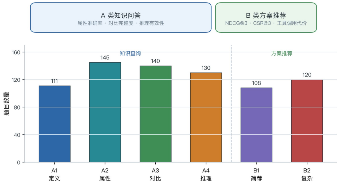
图 4 FWMAV-QA 数据集与评价协议
