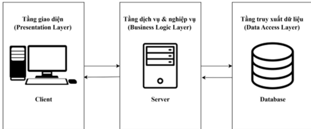
Hình 4.1. Sơ đồ mô tả kiến trúc logic hệ thống
