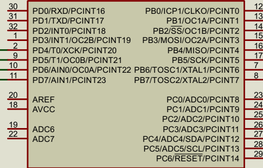
ATMEGA328P
