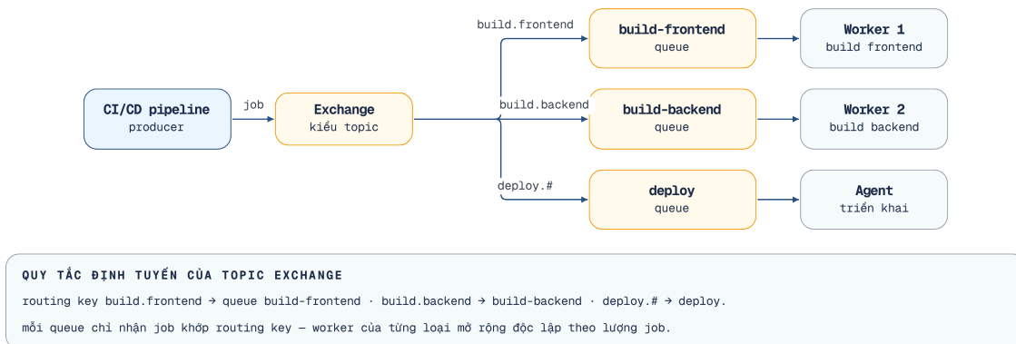
Hình 5.4: Kiến trúc RabbitMQ — Exchange định tuyến message đến các queue
