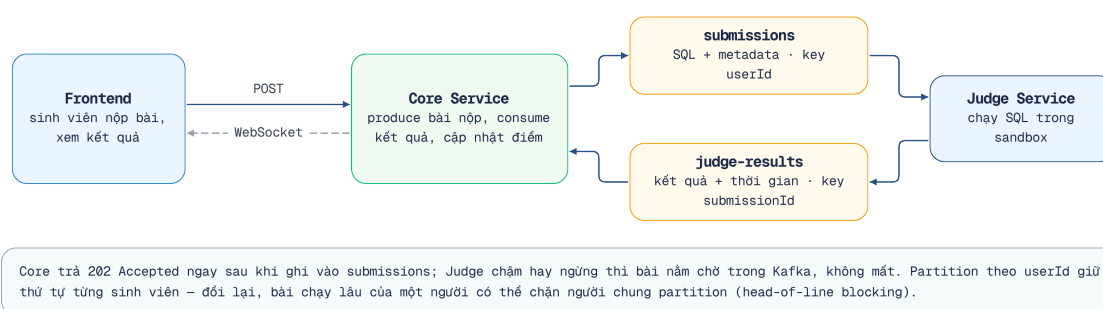
Hình 5.7: Kiến trúc pipeline 2 Kafka topic chấm bài trong chế độ thi
