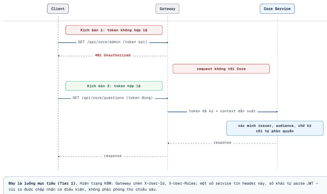
Hình 8.6: Luồng JWT tại Gateway — bằng chứng có chữ ký và context định danh dẫn xuất
