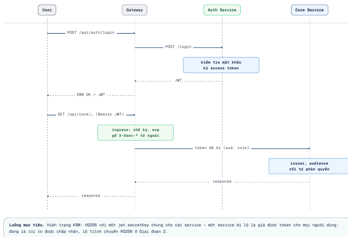
Hình 9.4: Luồng JWT mục tiêu — ingress validation, signed proof và local authorization
