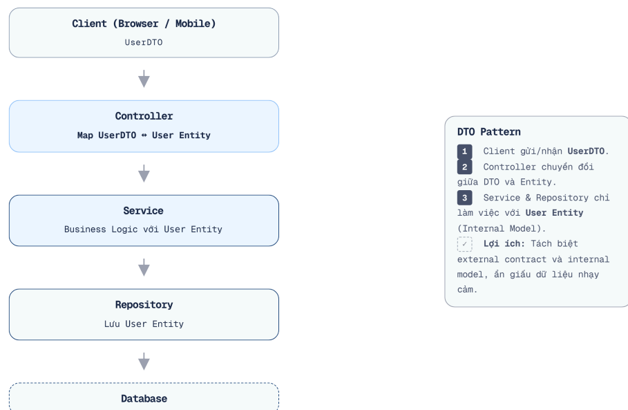
Hình 3.4: DTO pattern — tách internal model và external contract
