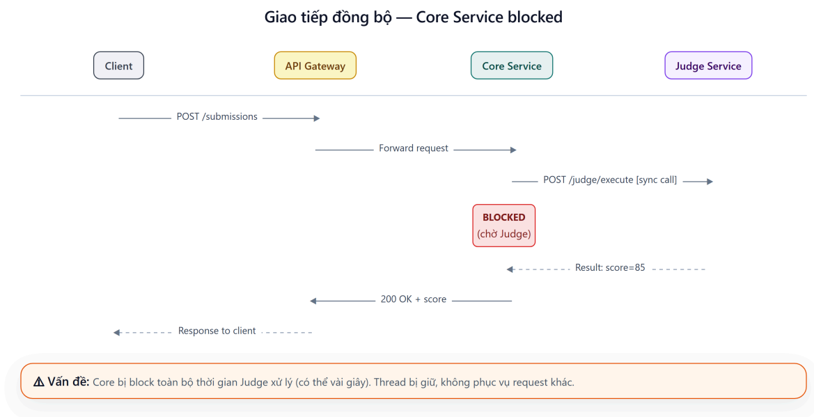
Hình 4.1: Giao tiếp đồng bộ — Core Service blocked trong khi chờ Judge response
