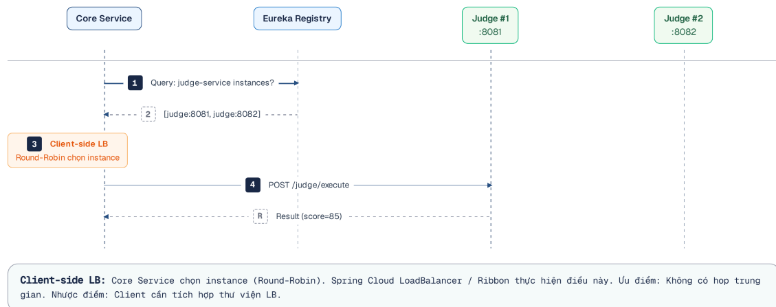
Hình 4.3: Client-side discovery — service tự query Eureka và load balance
