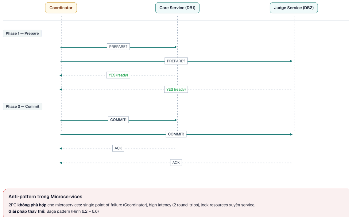
Hình 6.1: Two-Phase Commit — Coordinator điều phối prepare và commit
