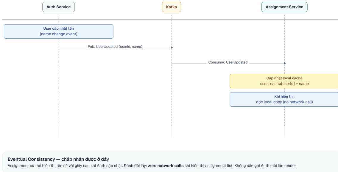
Hình 7.8: Truy cập dữ liệu xuyên service bằng Data Duplication qua Event Pipeline
