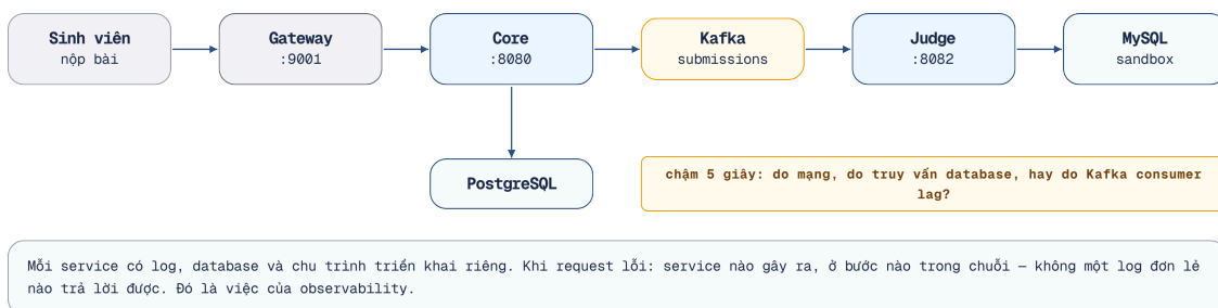
Hình 11.1: Luồng request qua 5+ services — lỗi xảy ra ở đâu?
