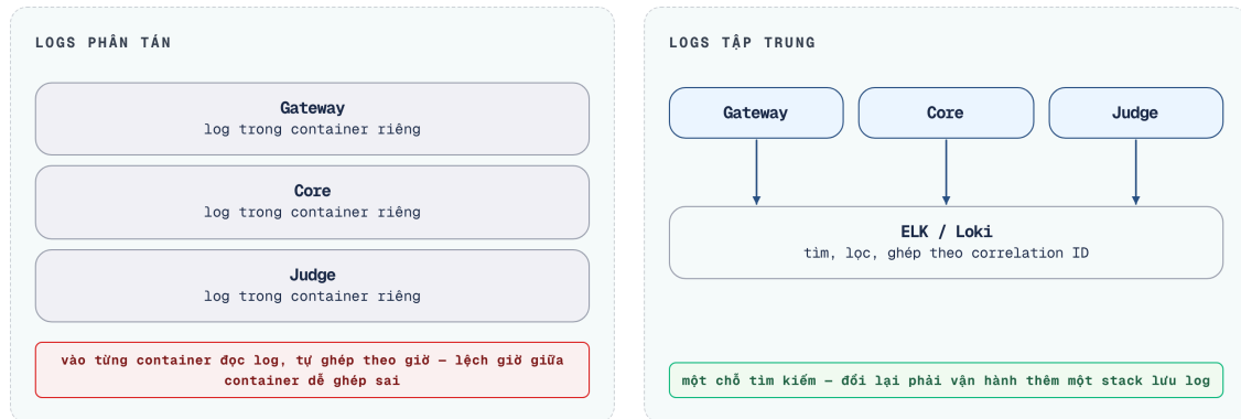
Hình 11.3: Logs phân tán (gỡ lỗi thủ công) vs Logs tập trung — tìm kiếm tại một nơi
